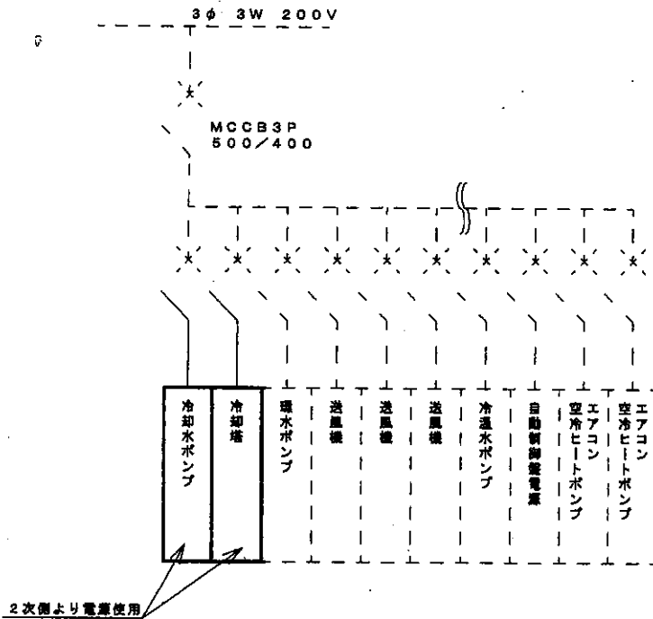
P-2 盤内
