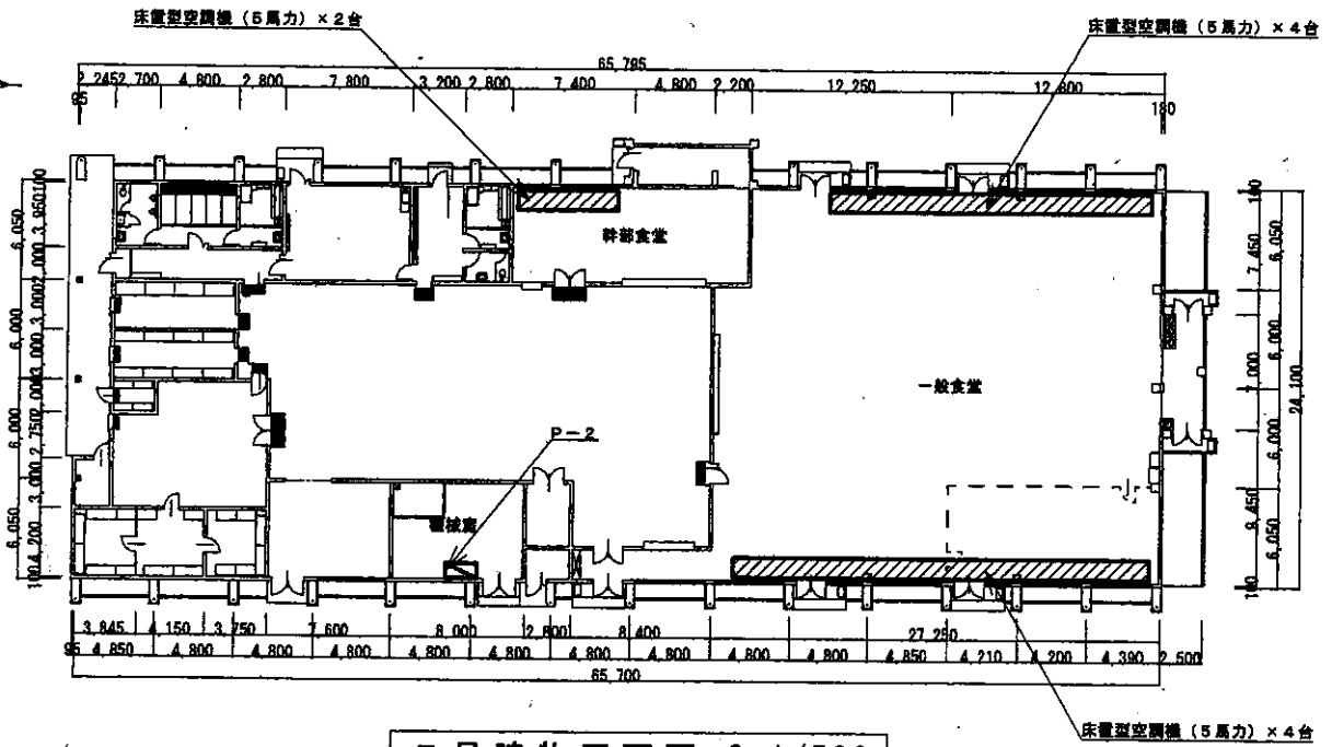
5号建物平面図 S=1/500
