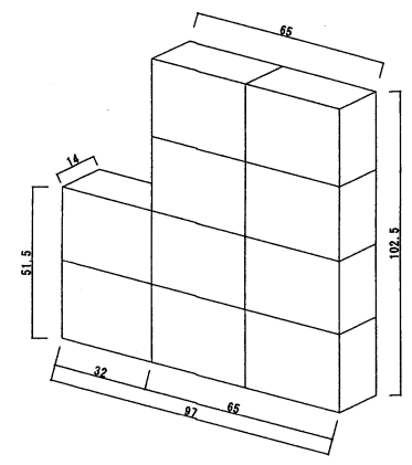
既設ポスト標準図 S=1/20
