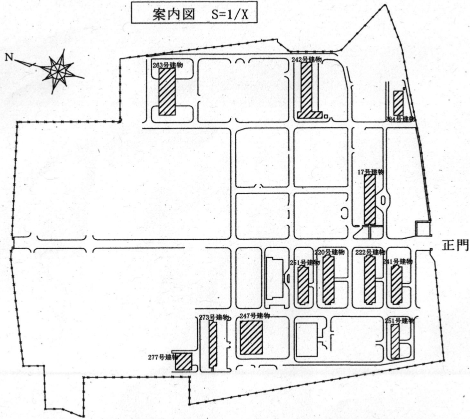
福岡駐屯地配置図 S=1/X
