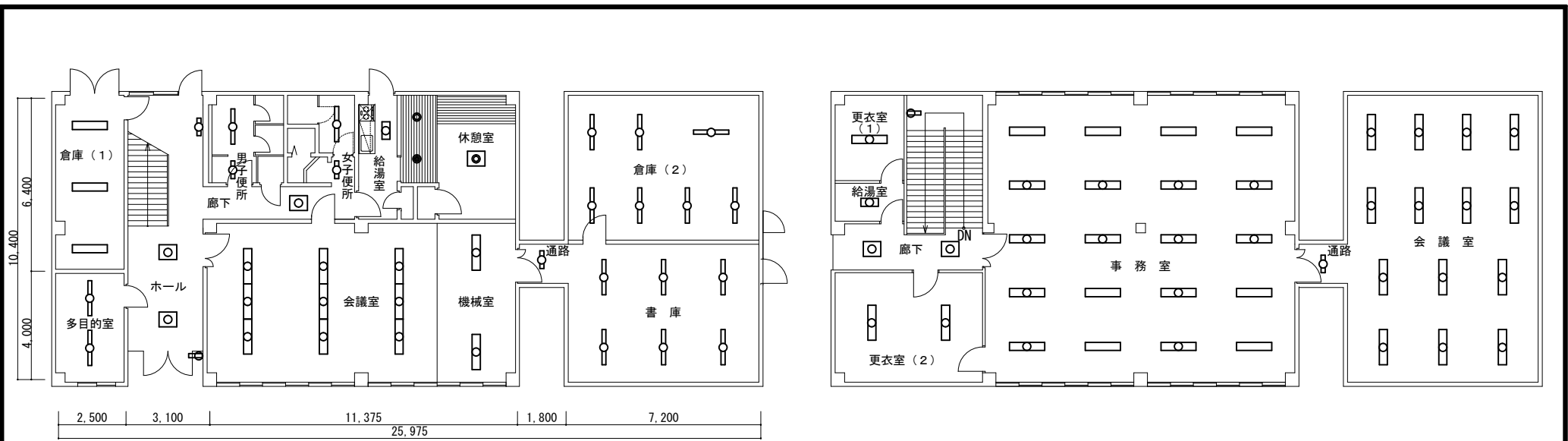
久留米地域事務所 電灯設備 1階平面図 1 / 150
