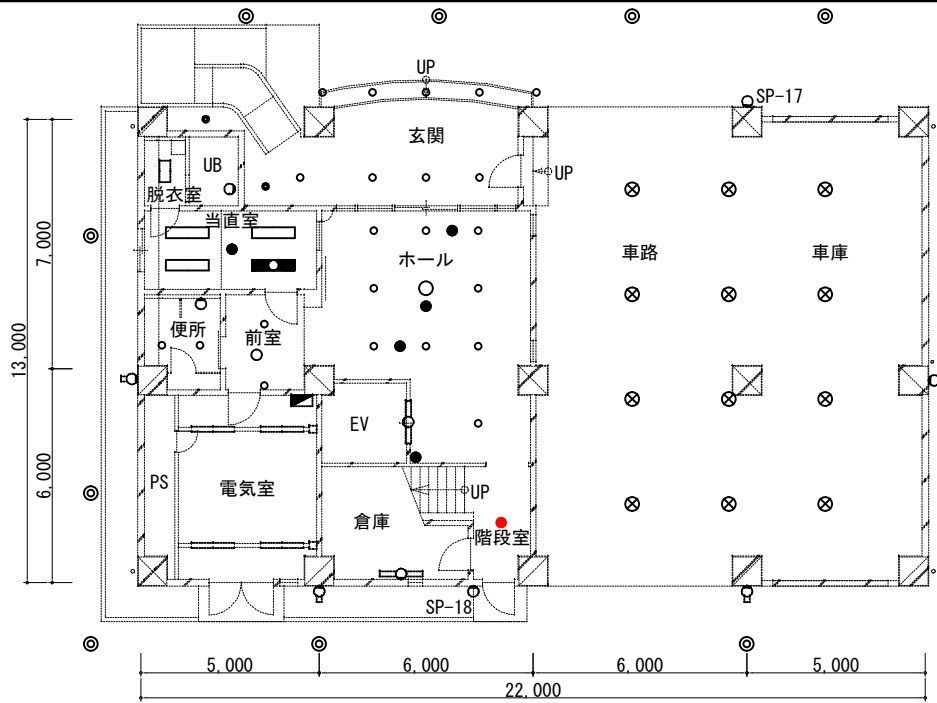
電灯設備 1階平面図 (改修前・改修後) 1 / 150
