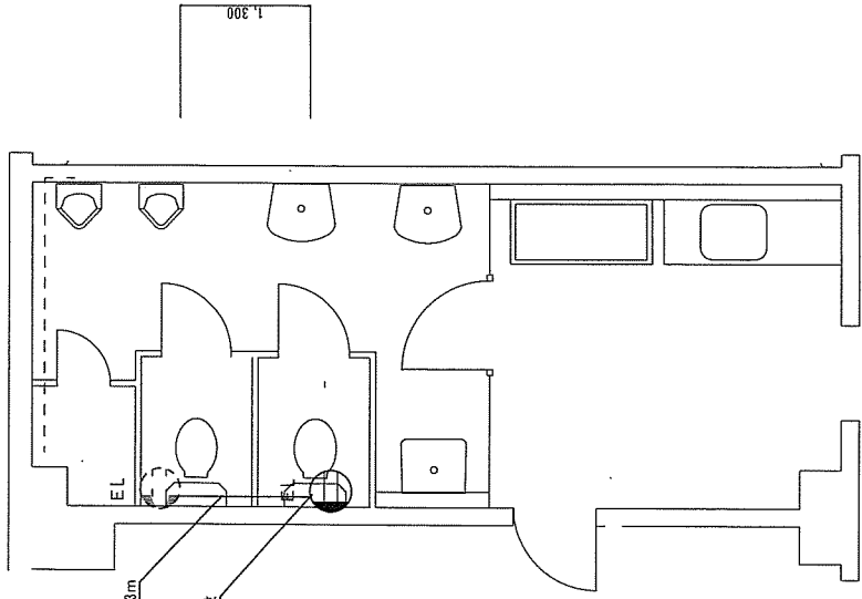
本部隊舎1階医務室トイレ改修後平面図 S=1/50
