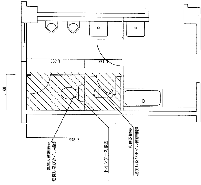
警衛所男子トイレ改修前平面図 S=1/50
