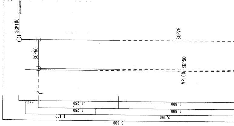
パイプシャフト通気管A面撤去立面図 S=1/25
