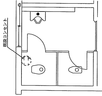
幹部隊舎トイレ改修前平面図 S=1/50
