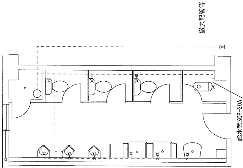
本部隊舎2階・3階男子トイレ改修前平面図 S=1/50
