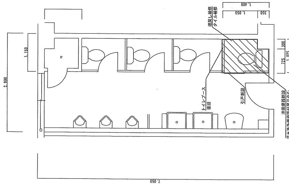
本部隊舎2階・3階男子トイレ改修後平面図 S=1/50
