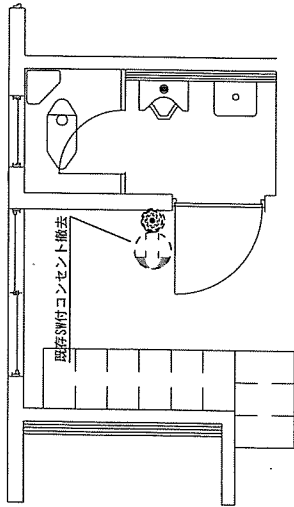
プール男子トイレ改修前平面図 S=1/50
