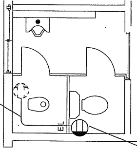
幹部隊舎トイレ改修後平面図 S=1/50
