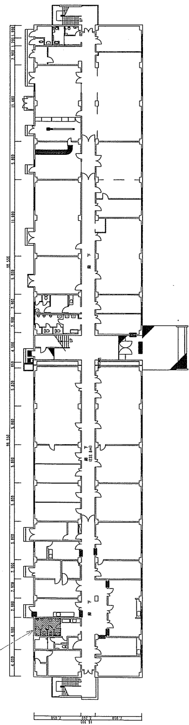
本部庁舎1階平面図 S=1/400
