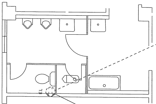
警衛所男子トイレ改修前平面図 S=1/50
