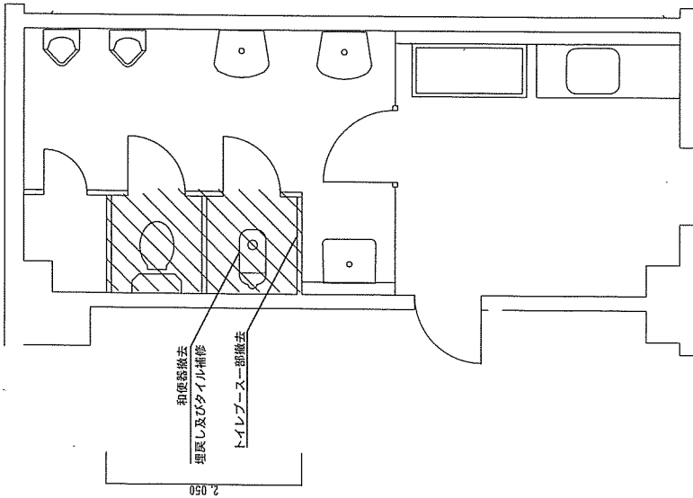
本部隊舎1階医務室トイレ改修前平面図 S=1/50
