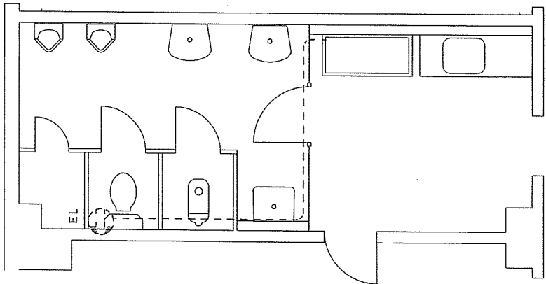
本部隊舎1階医務室トイレ改修前平面図 S=1/50
