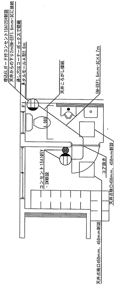
プール男子トイレ改修後平面図 S=1/50
