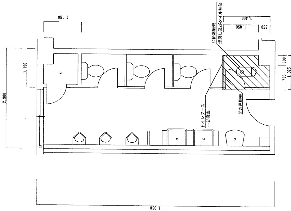
本部隊舎2階・3階男子トイレ改修前平面図 S=1/50
