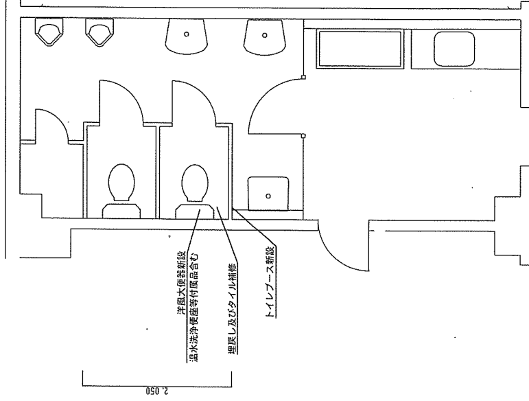
本部隊舎1階医務室トイレ改修後平面図 S=1/50
