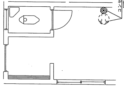
プール女子トイレ改修前平面図 S=1/50
