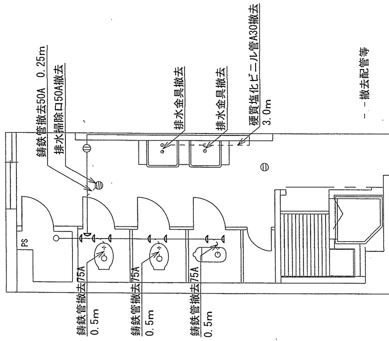
改修前排水設備平面図 S=1/50
