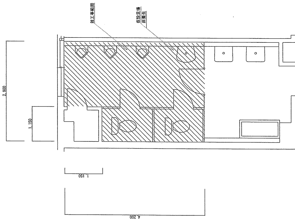
1階男子トイレ雑工事範囲 S=1/50
