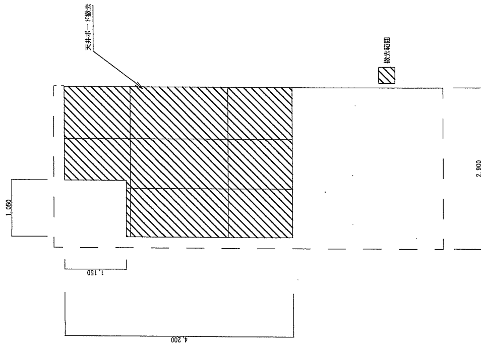
改修前天井伏図 S=1/50
