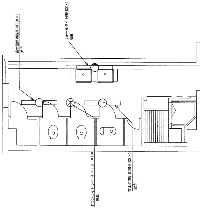
電灯設備 (既設)
