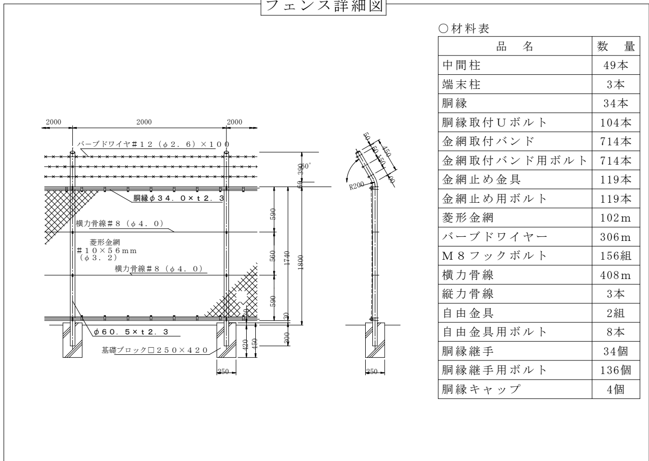
フェンス詳細図
