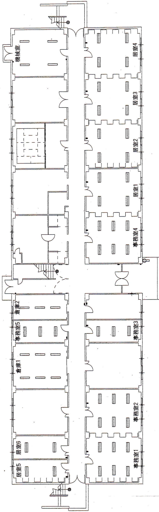
91号建物1階電灯設備図 S=1:200
