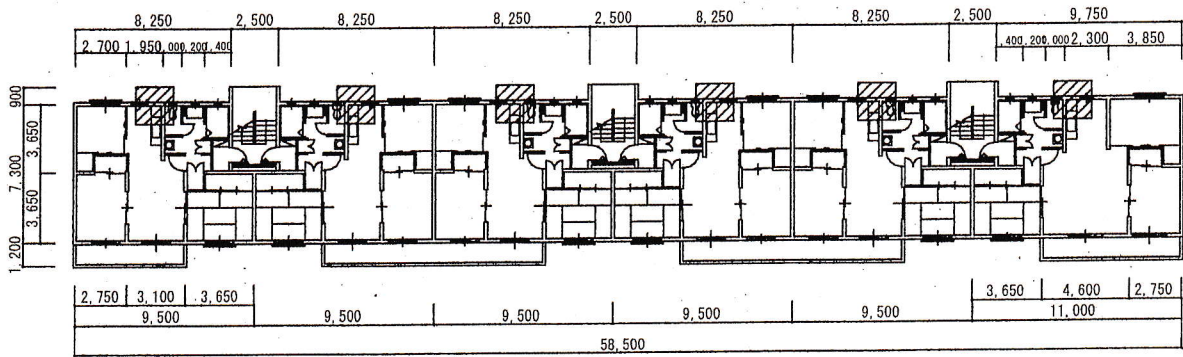
福島宿舎4号棟5階平面標準図 S=1/400 〇 施工箇所を示す
