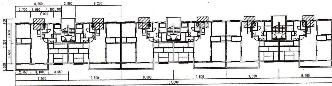
福島宿舎3号棟1階~5階平面標準図 S=1/400 〇 施工箇所を示す
