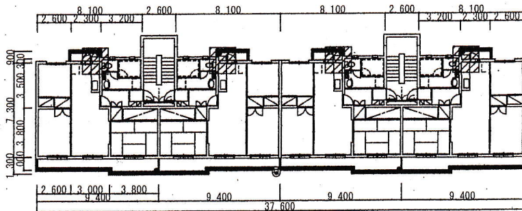
広瀬宿舎1階~5階平面標準図 S=1/400 〇 施工箇所を示す
