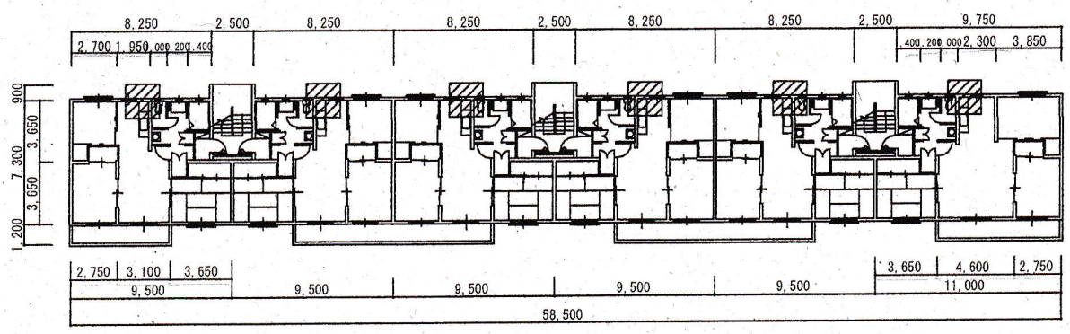
福島宿舎4号棟1階～4階平面標準図 S=1/400 施工箇所を示す
