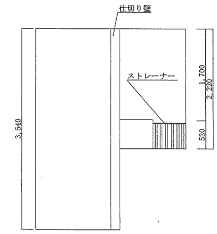
汚水中継槽 B-B' 面断面図
