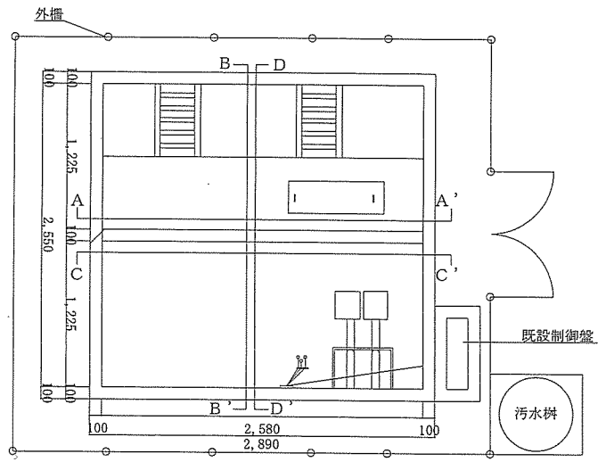
汚水中継槽平面図
