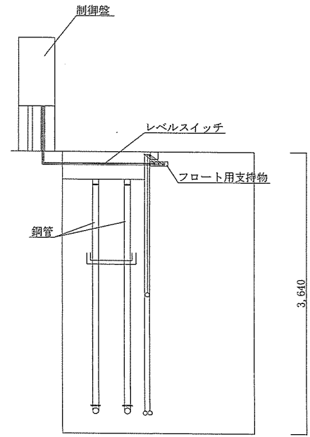
汚水中継槽 C-C' 面断面図
