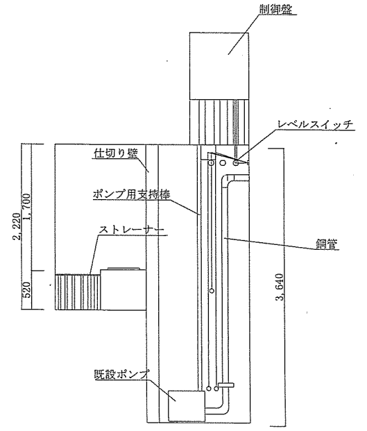
汚水中継槽 D-D' 面断面図
