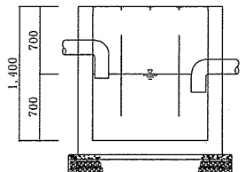
No.10油分離槽 S=1:70
