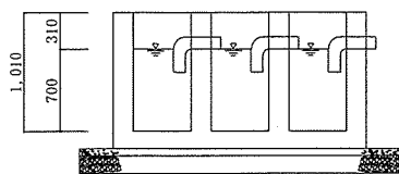
No.8油分離槽 S=1:70
