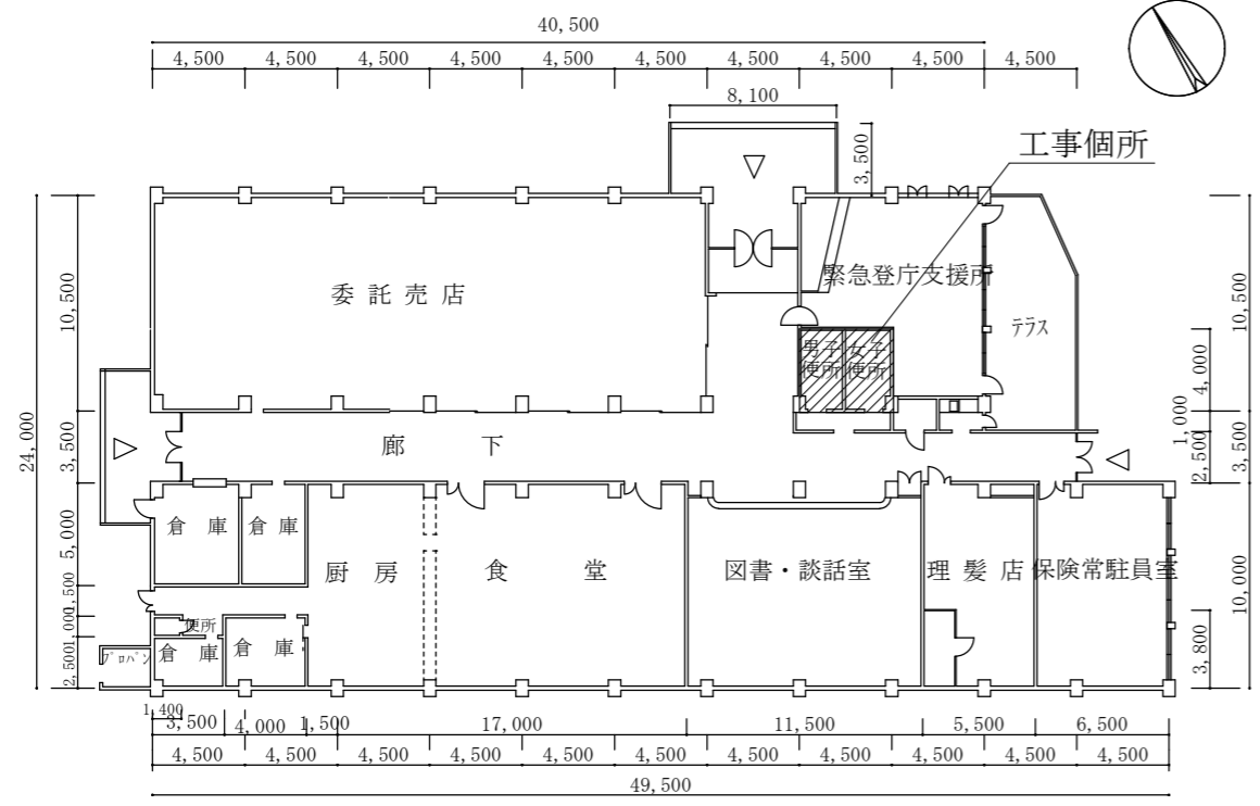
126号厚生センター平面図 1/400
