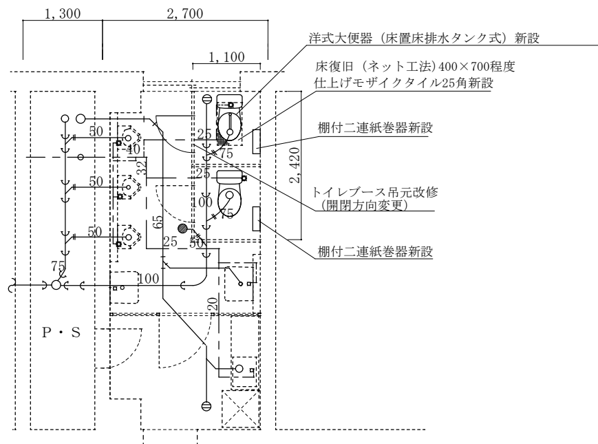
2階便所・湯沸室平面図 (改修後) 1/60
