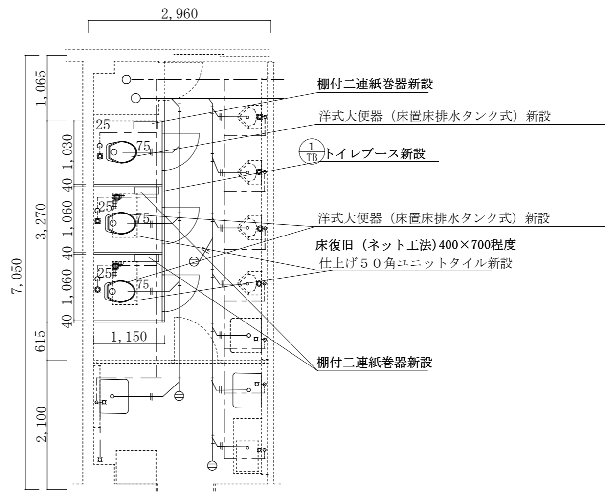
3号本部隊舎3階男子便所平面図 改修後 1/60
