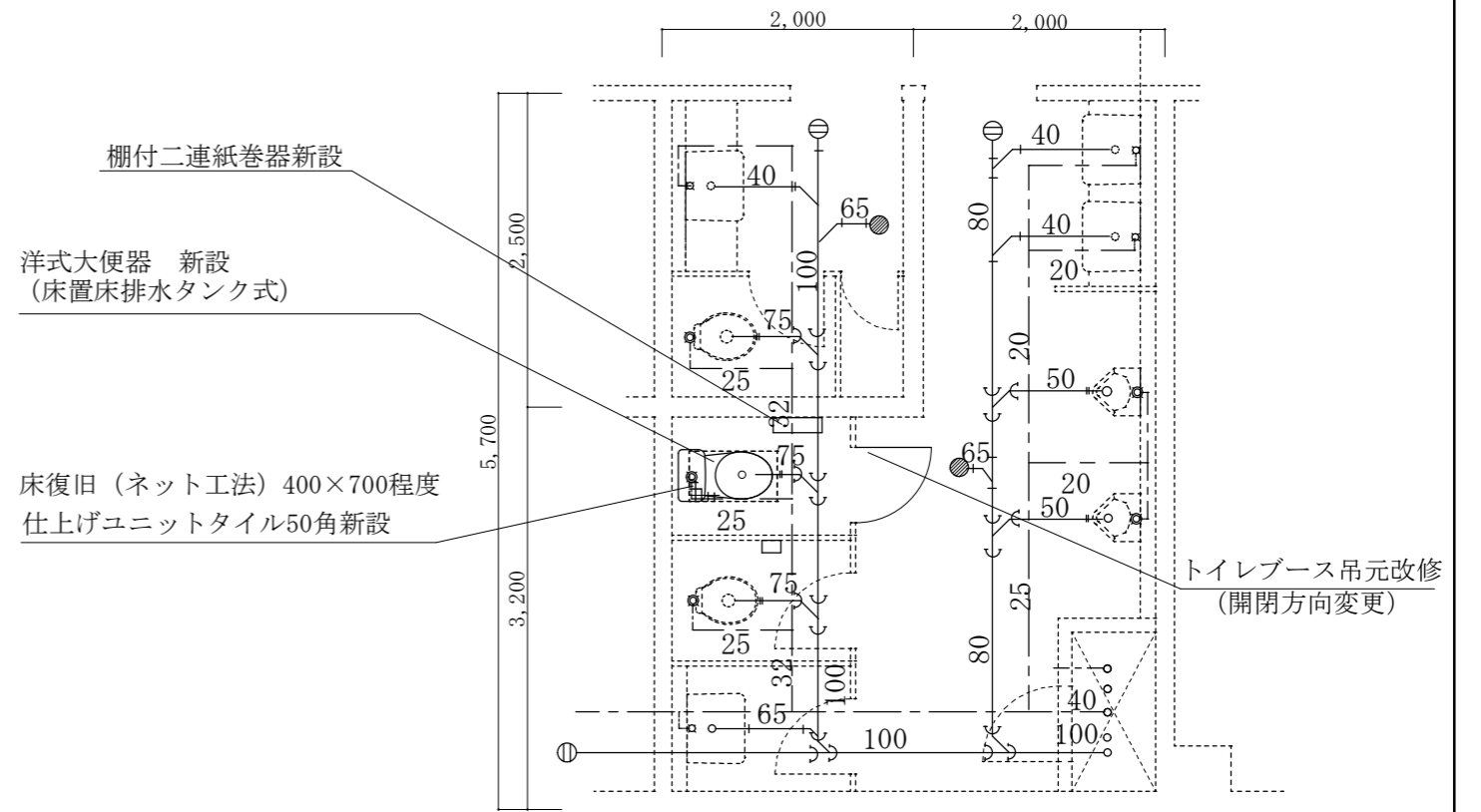
145号整備工場2階便所平面図 改修後 1/60
