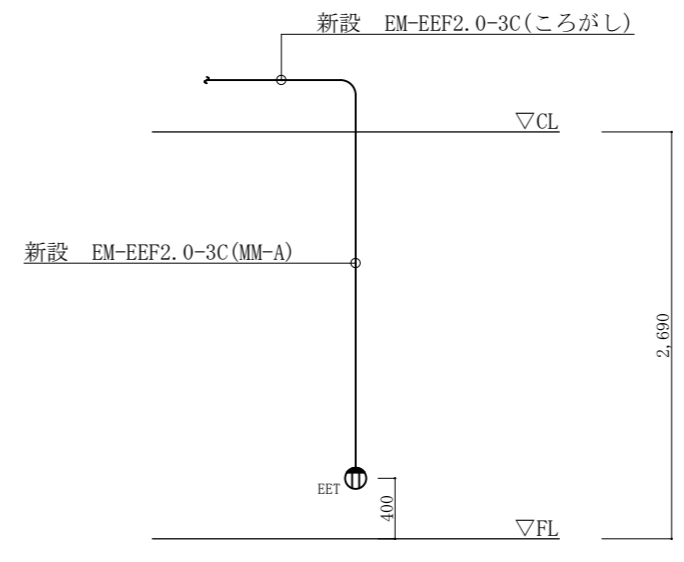
便座用コンセント取付正面図 (参考) S=1/50
