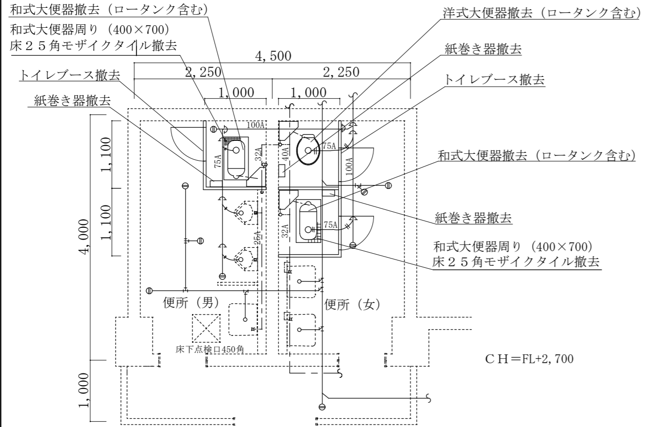
厚生センター便所平面図 (改修前) 1/60
