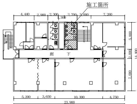
長崎合同庁舎 3階平面図 1/300
