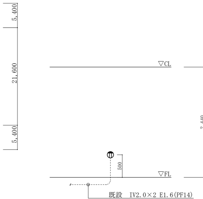
既存コンセント正面図 (改修前) S=1/50
