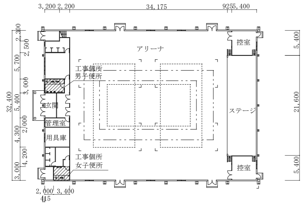
133号体育館平面図 1/500
