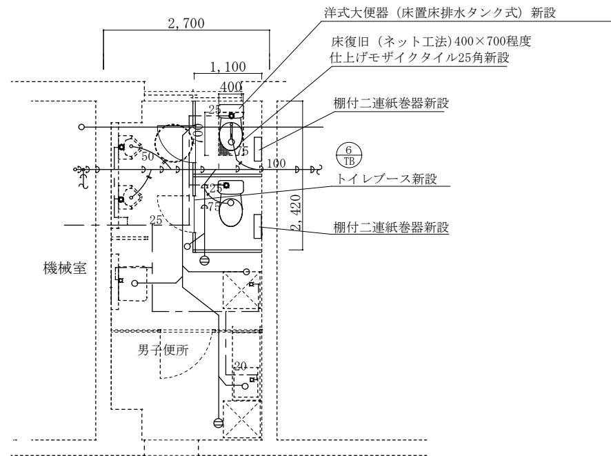
1階便所・湯沸室平面図 (改修後) 1/60
