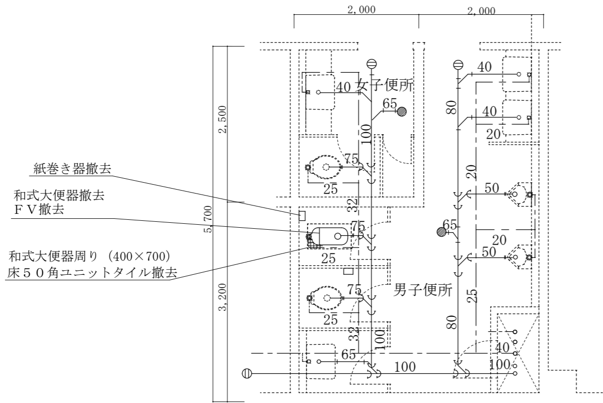
145号整備工場2階便所平面図 改修前 1/60
