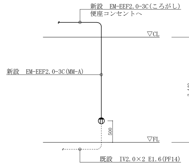
既存コンセント正面図 (改修後) S=1/50
