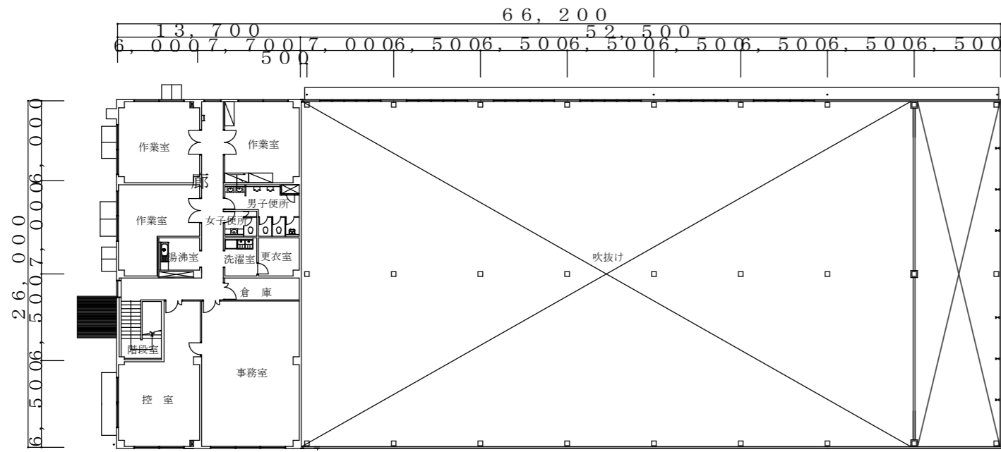
145号整備工場2階平面図 1/400
