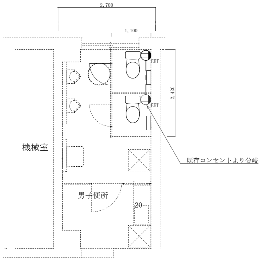
1階便所・湯沸室 コンセント設備平面図 (改修後) S=1/60
