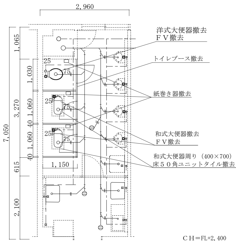
3号本部隊舎3階男子便所平面図 改修前 1/60
