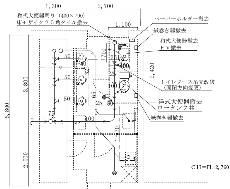
3階便所・湯沸室平面図 (改修前) 1/60
