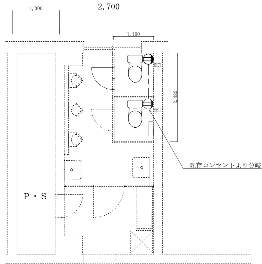
2階便所・湯沸室 コンセント設備平面図 (改修後) S=1/60
