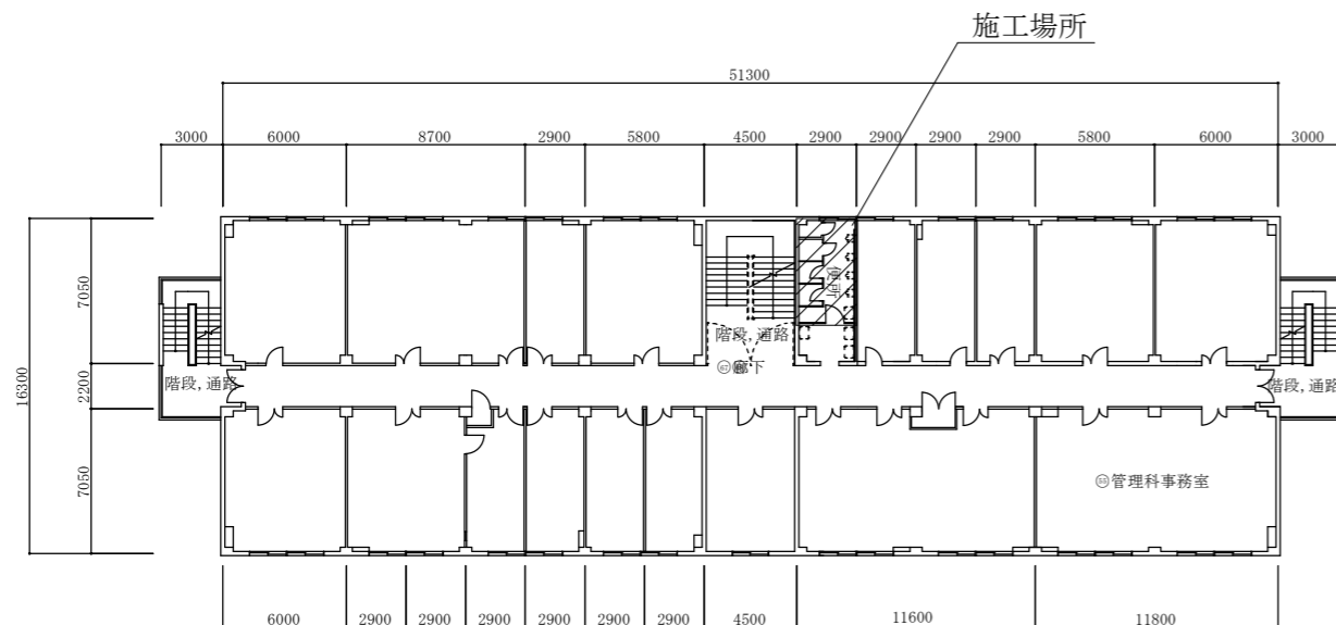
3号本部隊舎3階平面図 S=1/400
