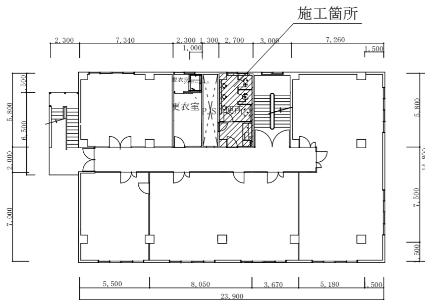
長崎合同庁舎 2階平面図 S=1/400
