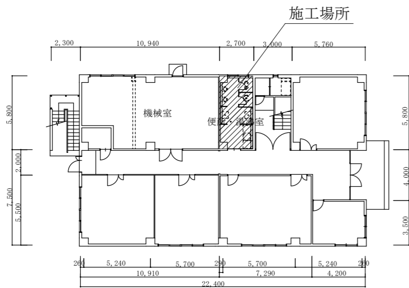
長崎合同庁舎 1階平面図 S=1/400
