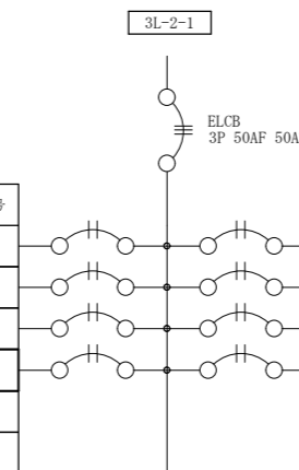
3号電灯分電盤結線図 (改修後) S=NONE
