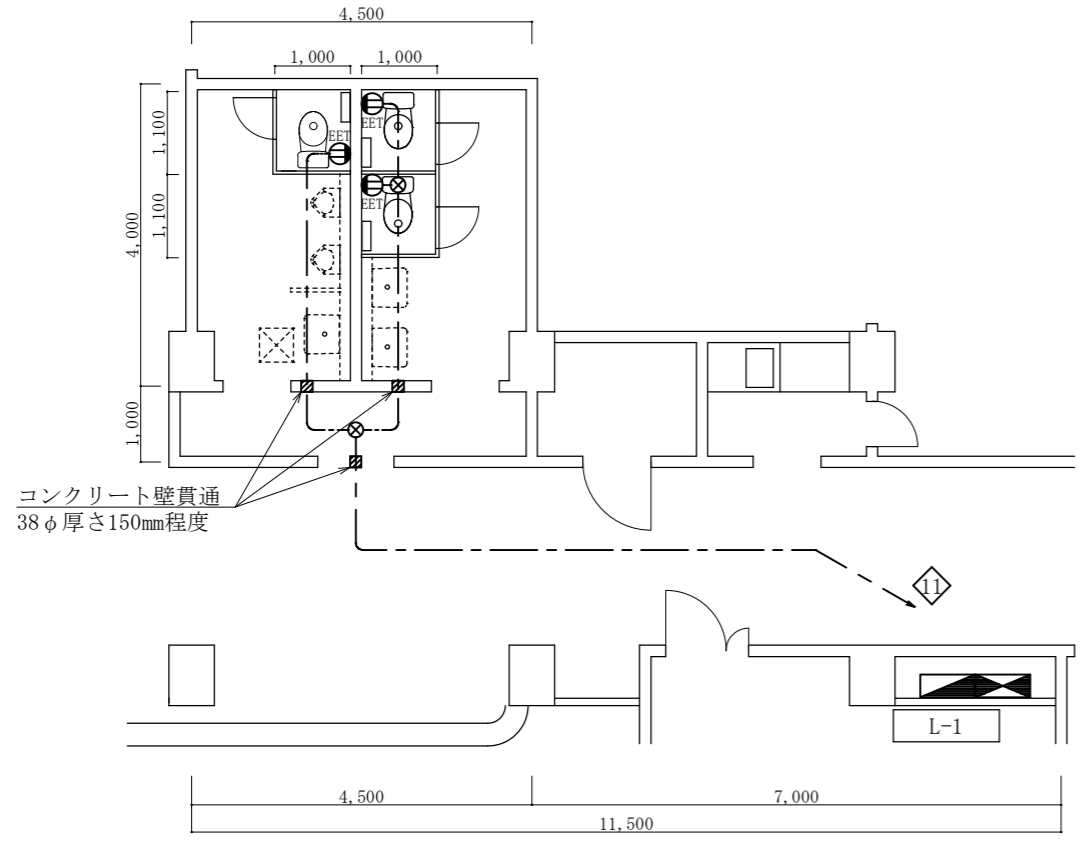
126号コンセント設備平面図 (改修後) S=1/100
