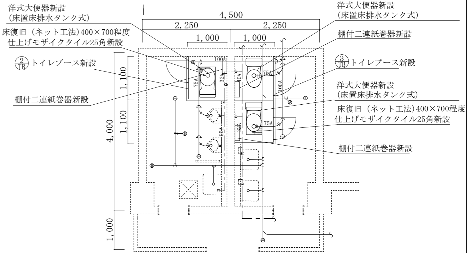
厚生センター便所平面図 (改修後) 1/60
