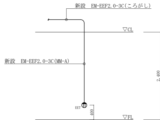
便座用コンセント取付正面図 (参考) S=1/50
