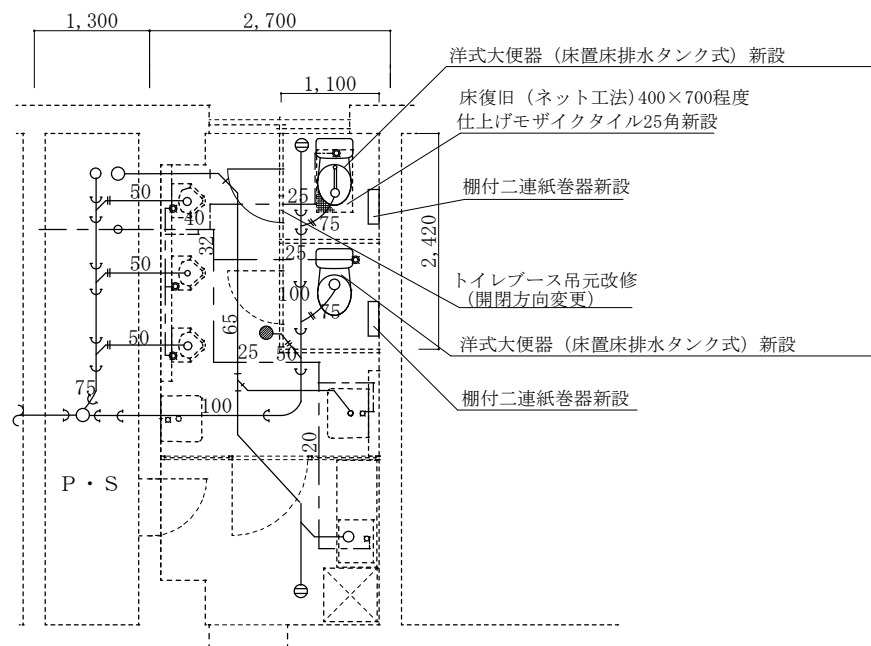
3階便所・湯沸室平面図 (改修後) 1/60
