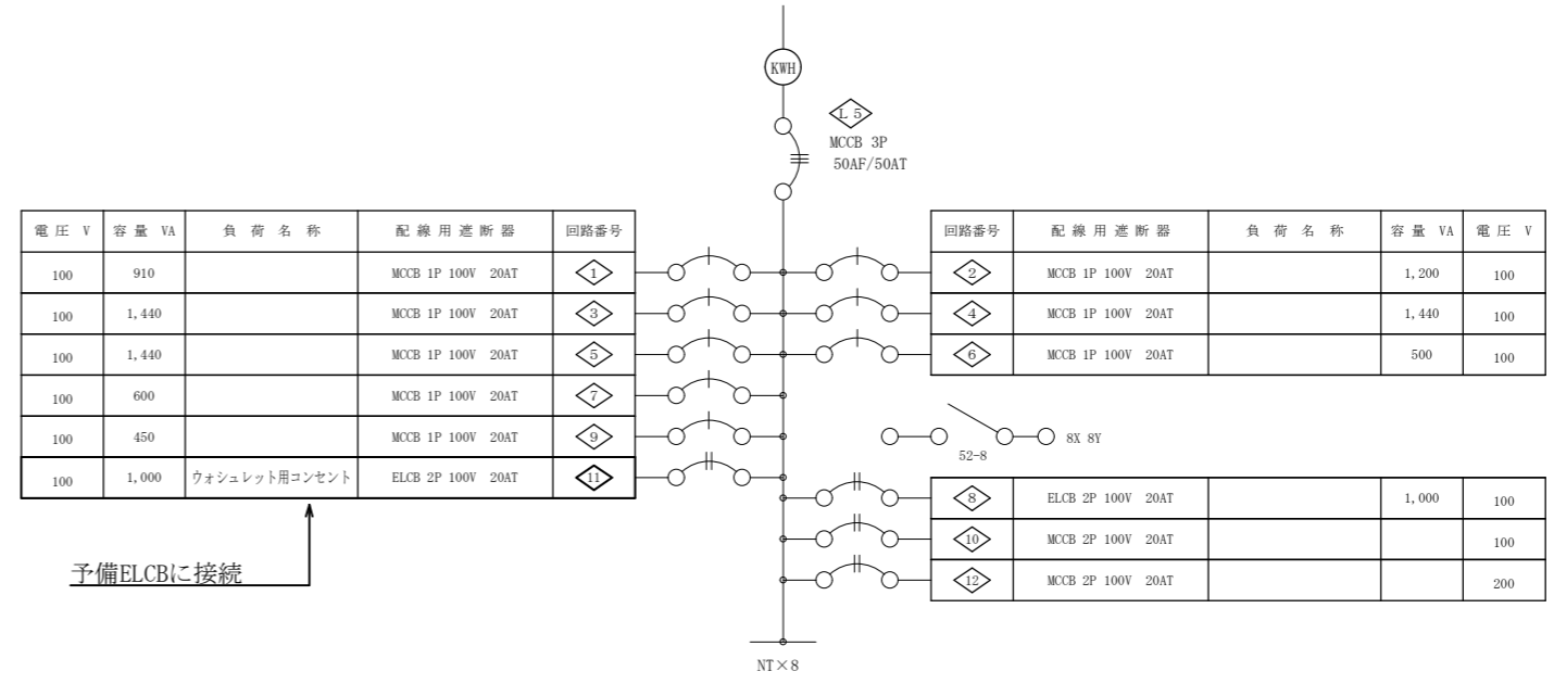
126号電灯分電盤結線図 (改修後) S=NONE
