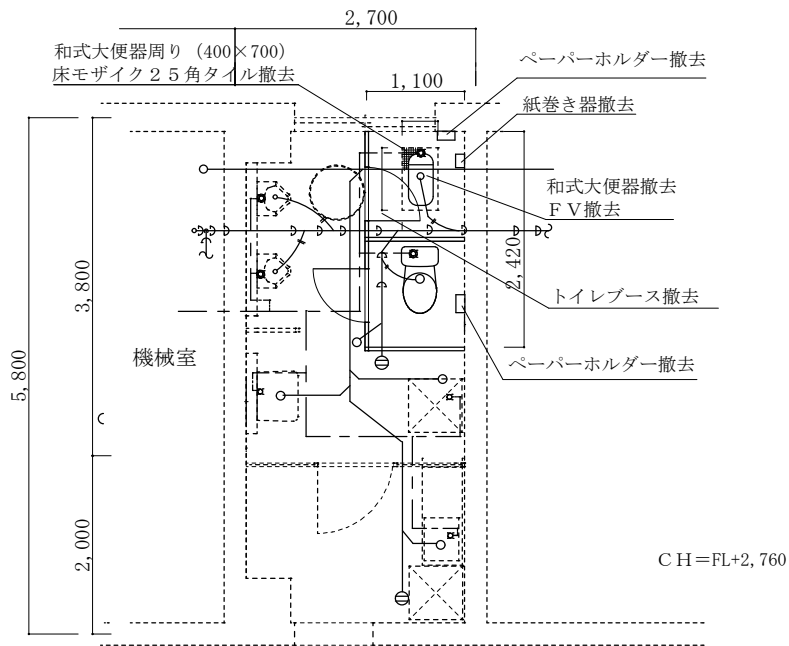
1階便所・湯沸室平面図 (改修前) 1/60
