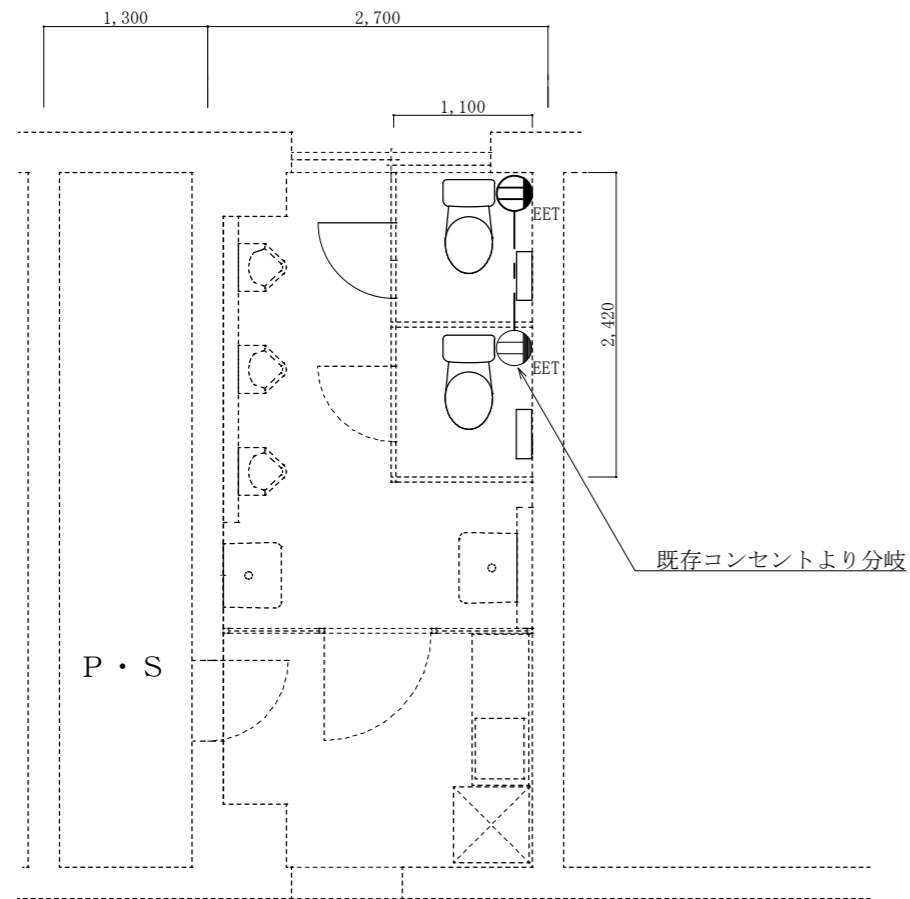
3階便所・湯沸室 コンセント設備平面図 (改修後) S=1/60
