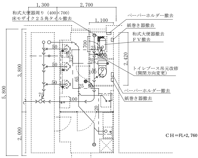
2階便所・湯沸室平面図 (改修前) 1/60
