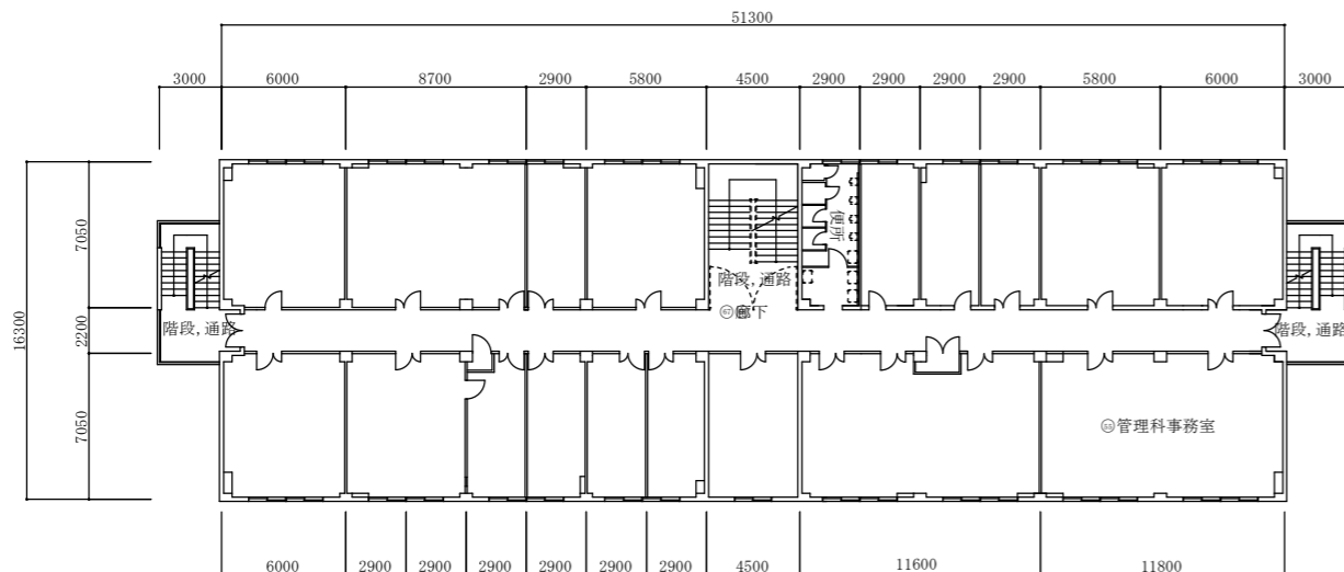
3号本部隊舎3階平面図 1/400
