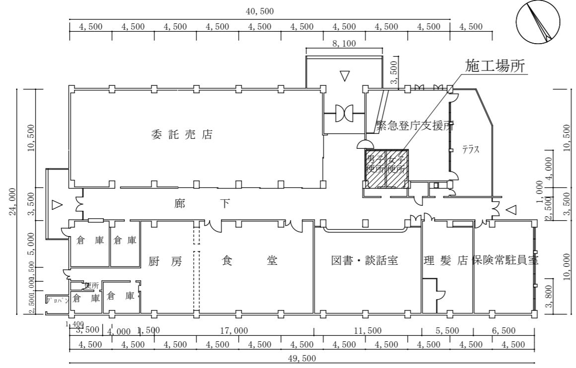
126号厚生センター平面図 S=1/400
