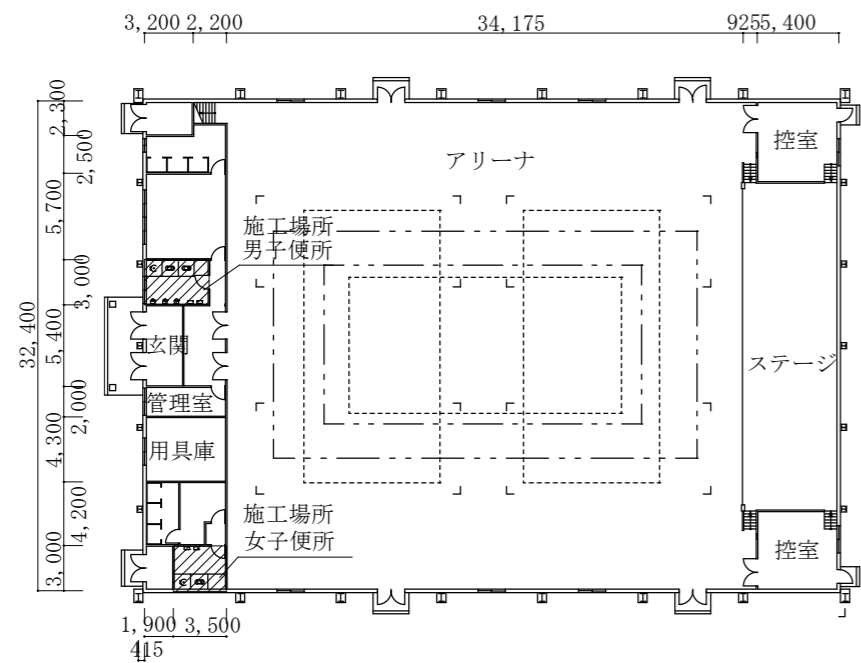
133号体育館平面図 S=1/500
