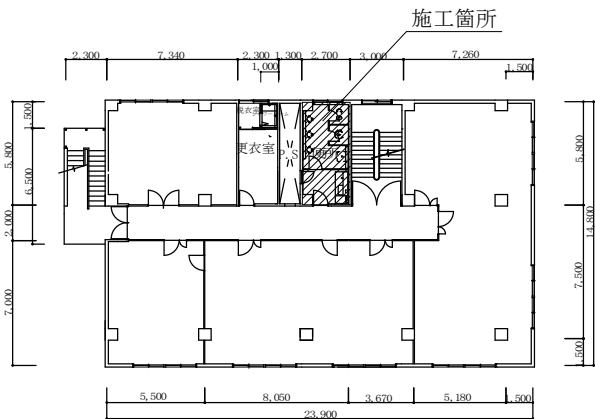
長崎合同庁舎2階平面図 1/300
