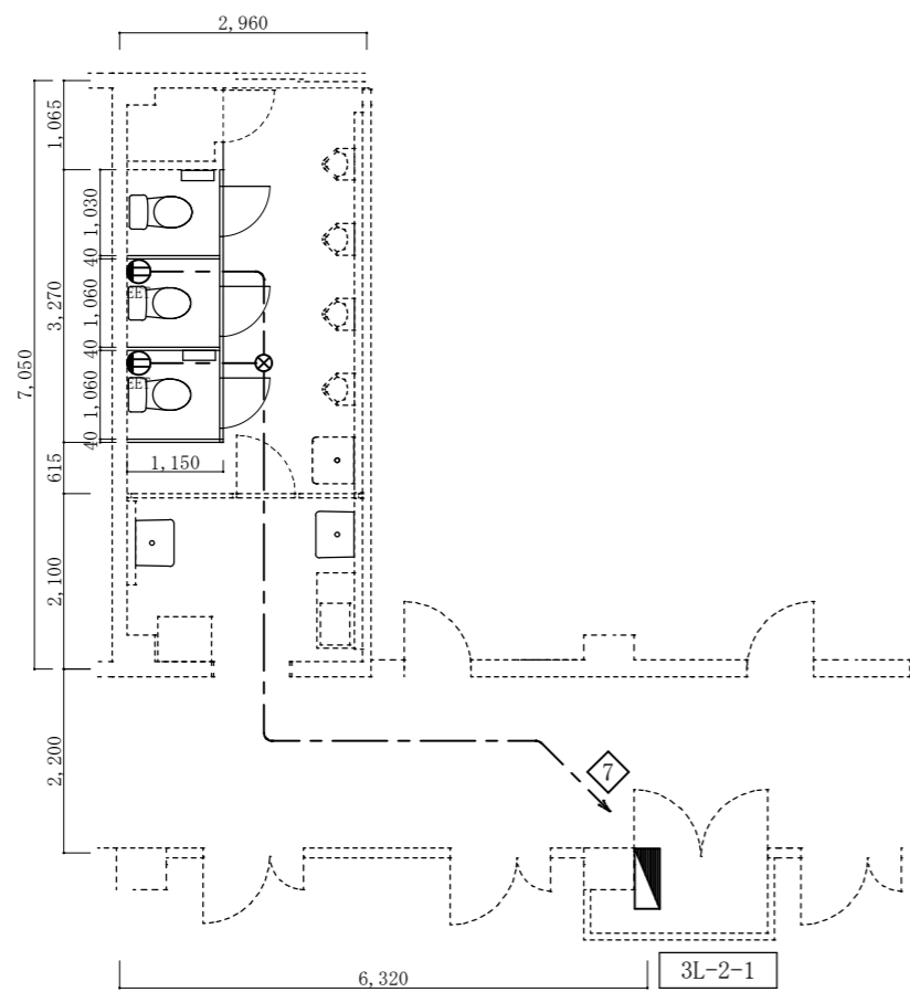
3号3階コンセント設備平面図 (改修後) S=1/100
