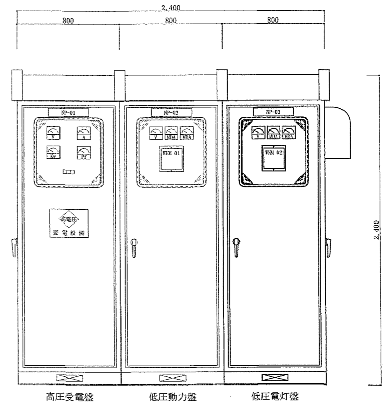
8号建物変電設備 立面図 S=1:30
