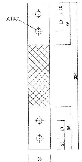
8号建物変電設備 立面図 S=1:30
