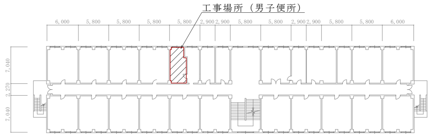
1階平面図 S=1:450
