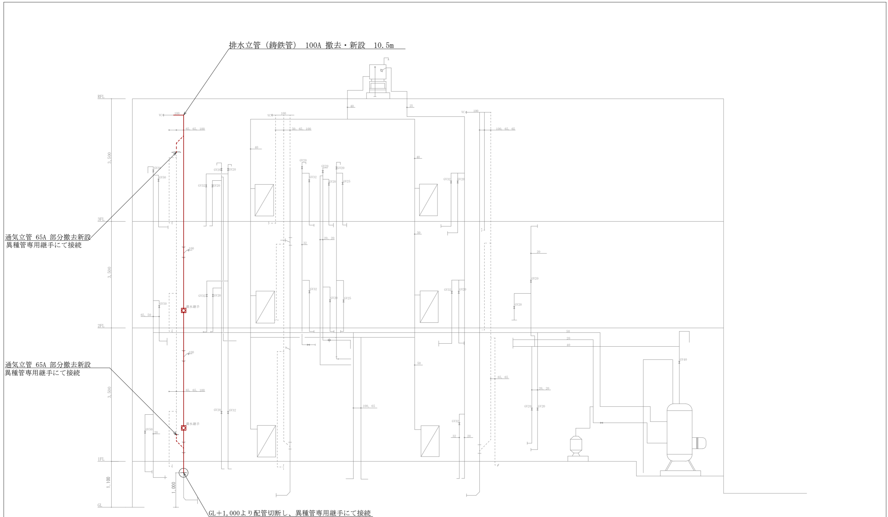
衛生設備配管系統図
