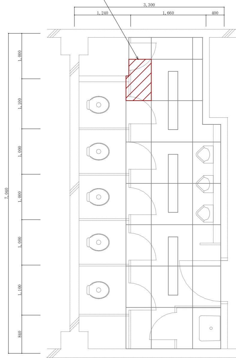
2階天井伏図 S=1:50
