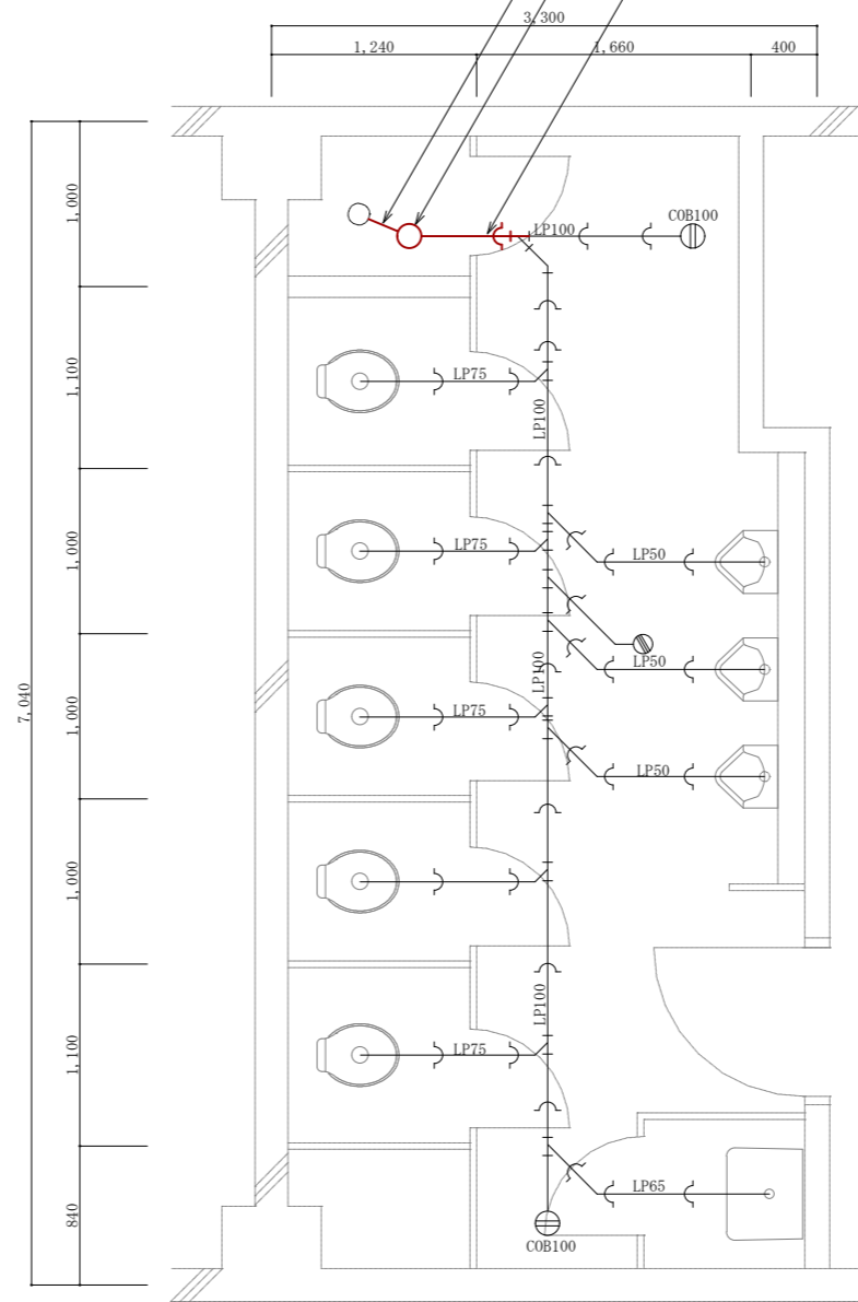
3階排水管系統図 S=1:50
