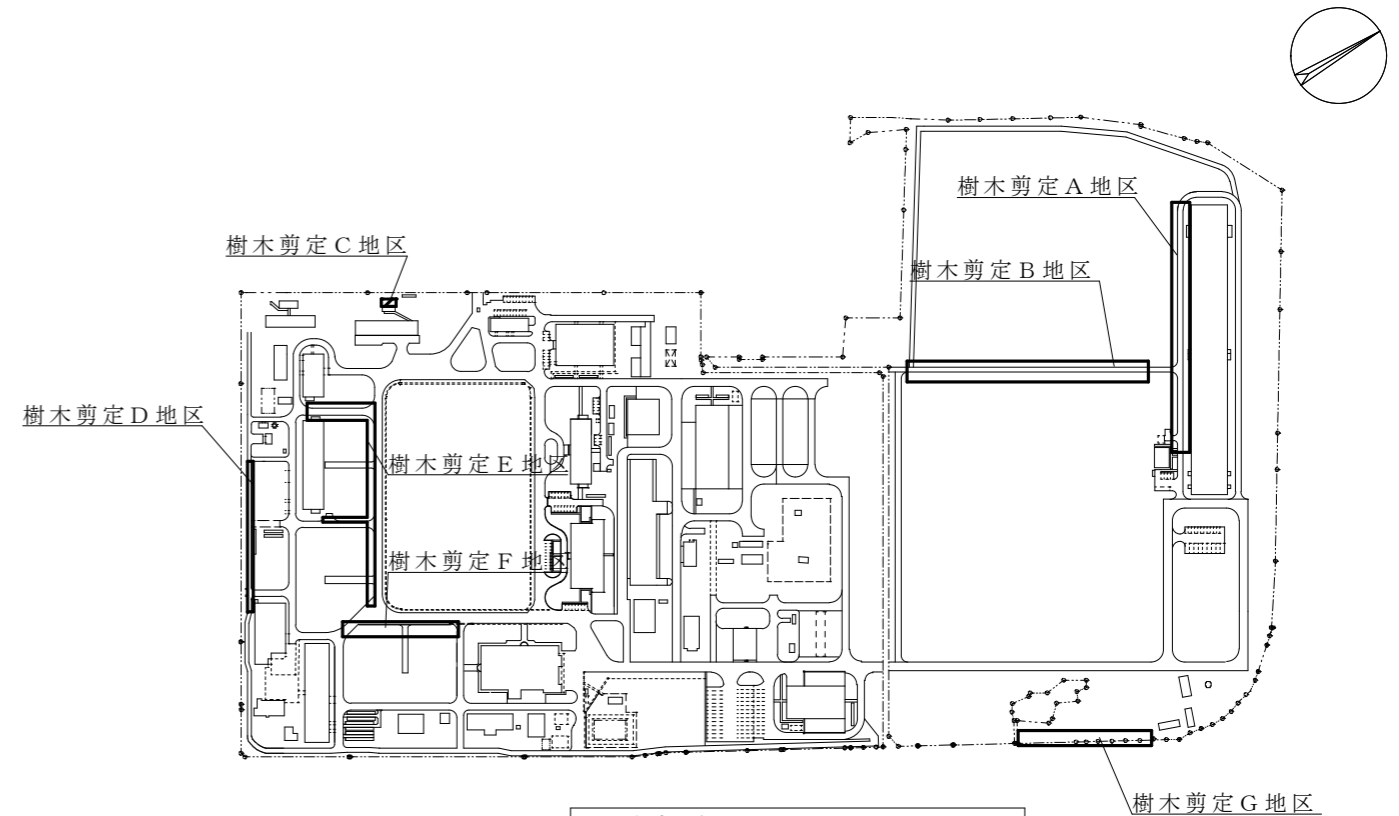
大村駐屯地配置図 S=1:X
