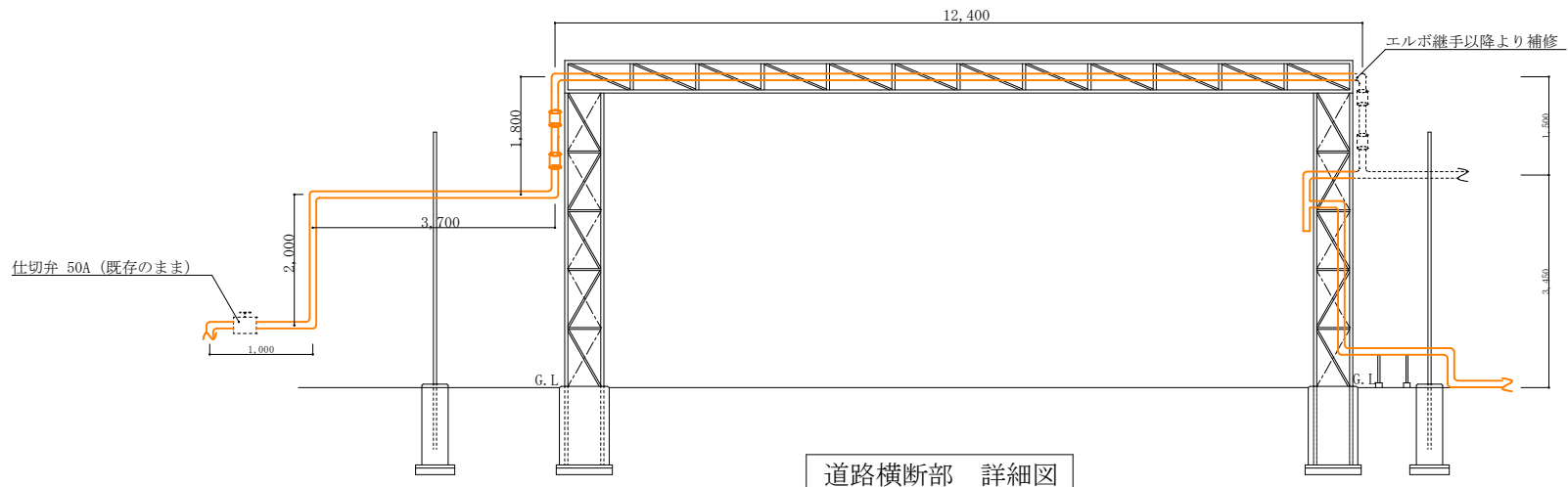
施工平面図 S=1:350
