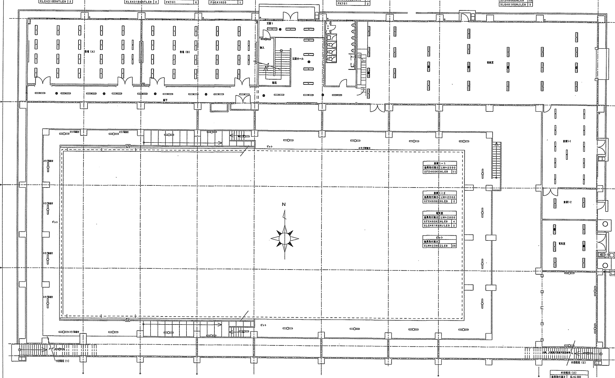
148号訓練場1階 電灯設備平面図
