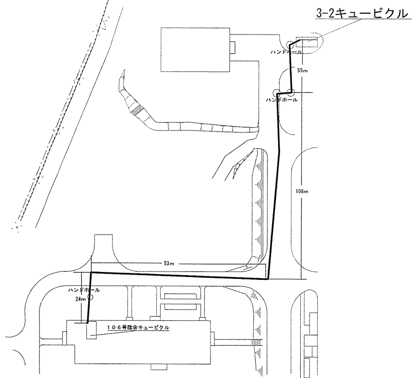
ケーブル更新図 S=1/X
