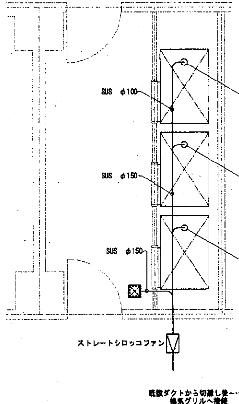
シャワー室換気設備平面図 S=1/60
