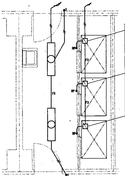
シャワー室照明設備平面図 S=1/60
