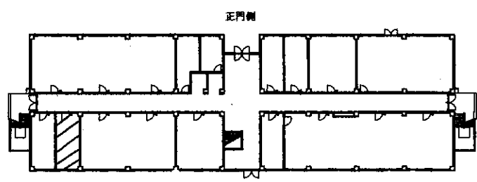
128号隊舎 1階平面図
