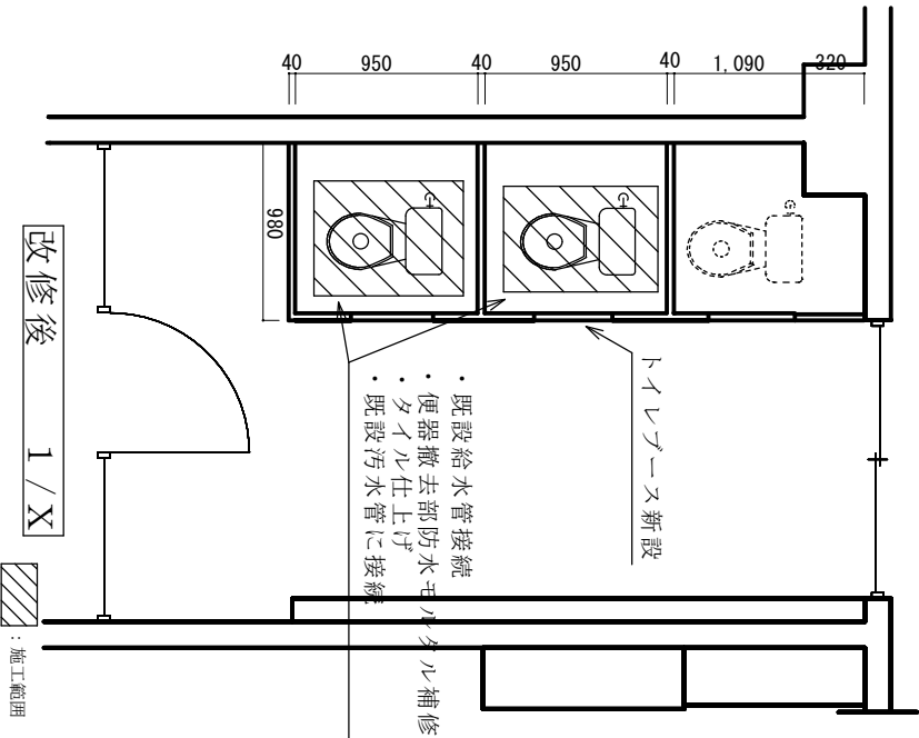
100号建物 1F平面図
