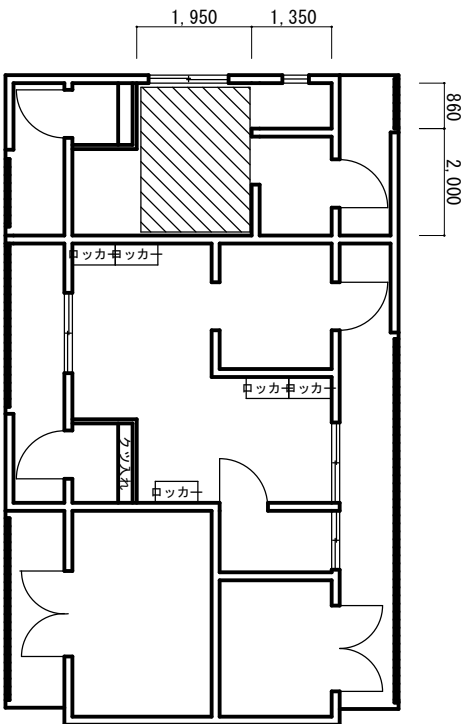
プール管理棟平面図
