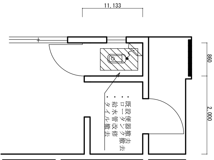
プール女子便所改修前 1/X
