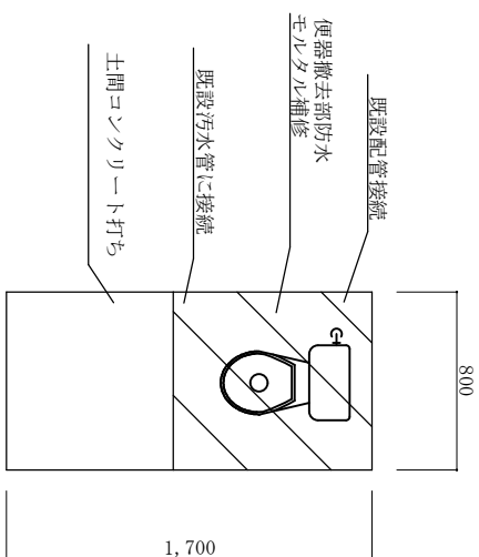
86号建物女子便所改修後平面図
