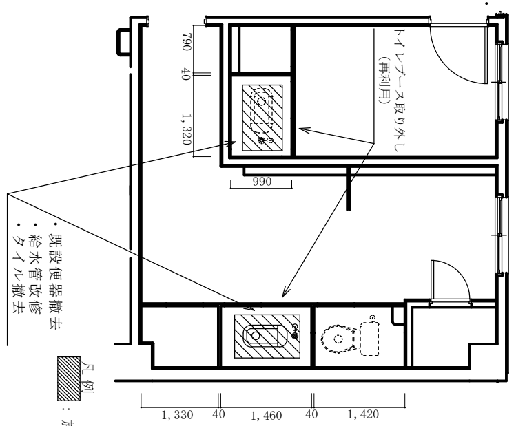
便所改修前平面図 1/X
