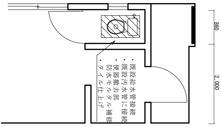
プール女子便所改修後 1/X
