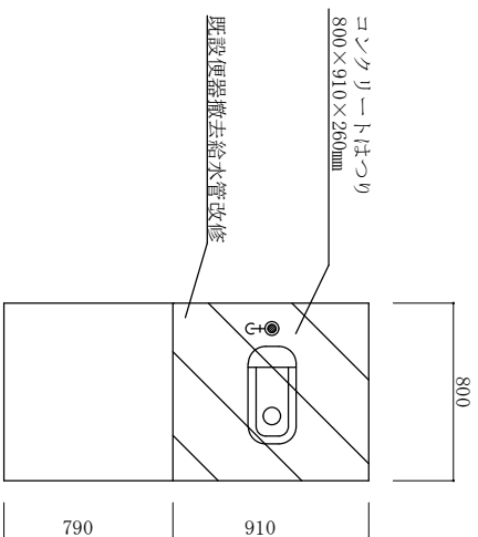
86号建物女子便所改修前平面図
