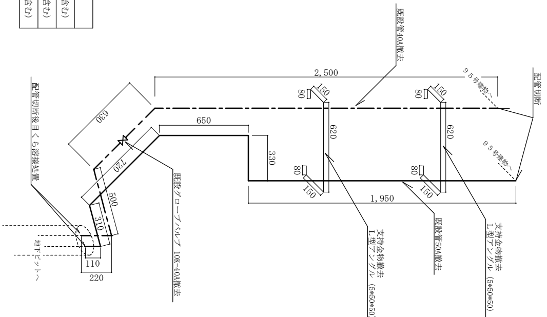
蒸気管平面図 B部撤去詳細図
