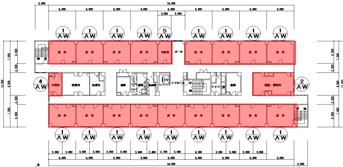
4階平面図（20台）
