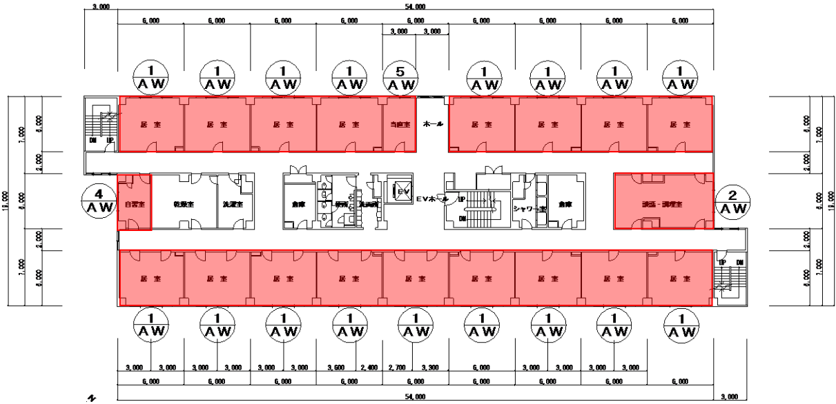
5階平面図（20台）
