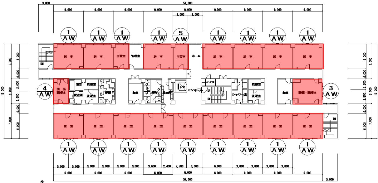
6階平面図（20台）
