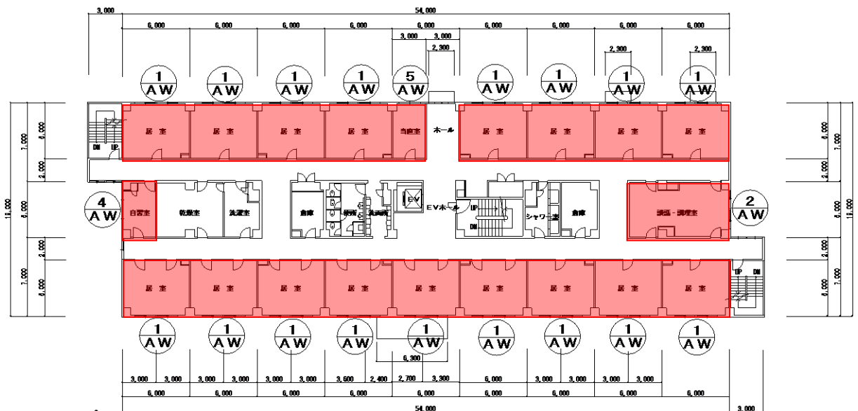
2階平面図 (20台)
