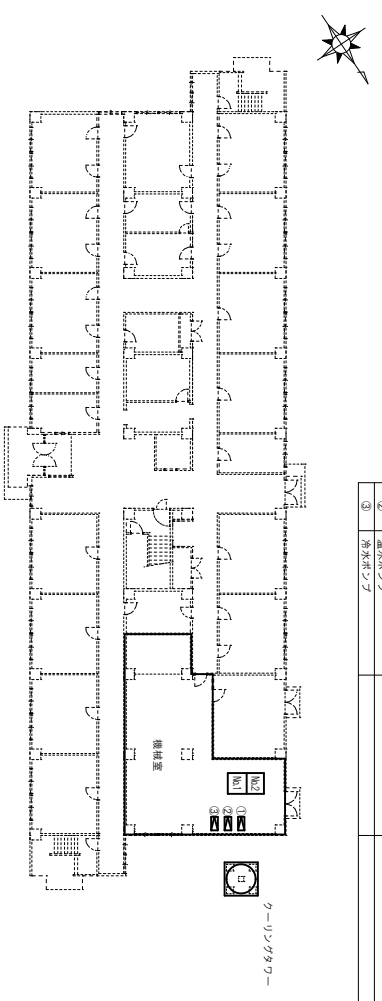
才 4号隊舎1階機器配置図 S=1/400
