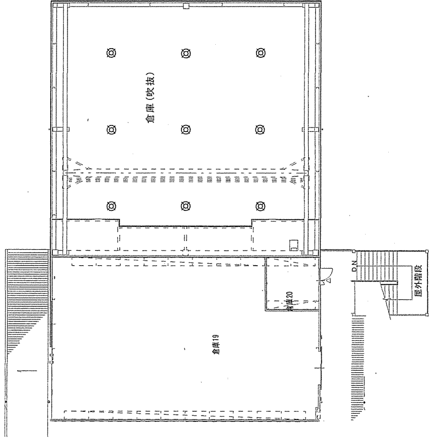
136号建物東側倉庫電灯設備図 S=1:200
