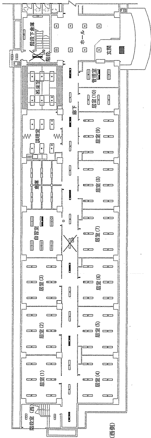
116号建物1階電灯設備図 S=1:200
