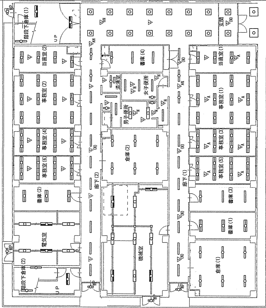
1 2 5 号建物 1 階西側電灯設備図 S=1:175
