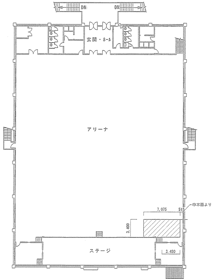
体育館（2F）床板補修施工平面図 S=1/300
