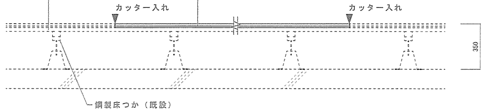
体育館（2F）床板補修施工断面図 S=1/20
