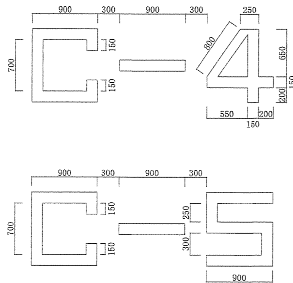
駐機円英数字詳細図 S=1:50 ※白線 実線 幅15cm
