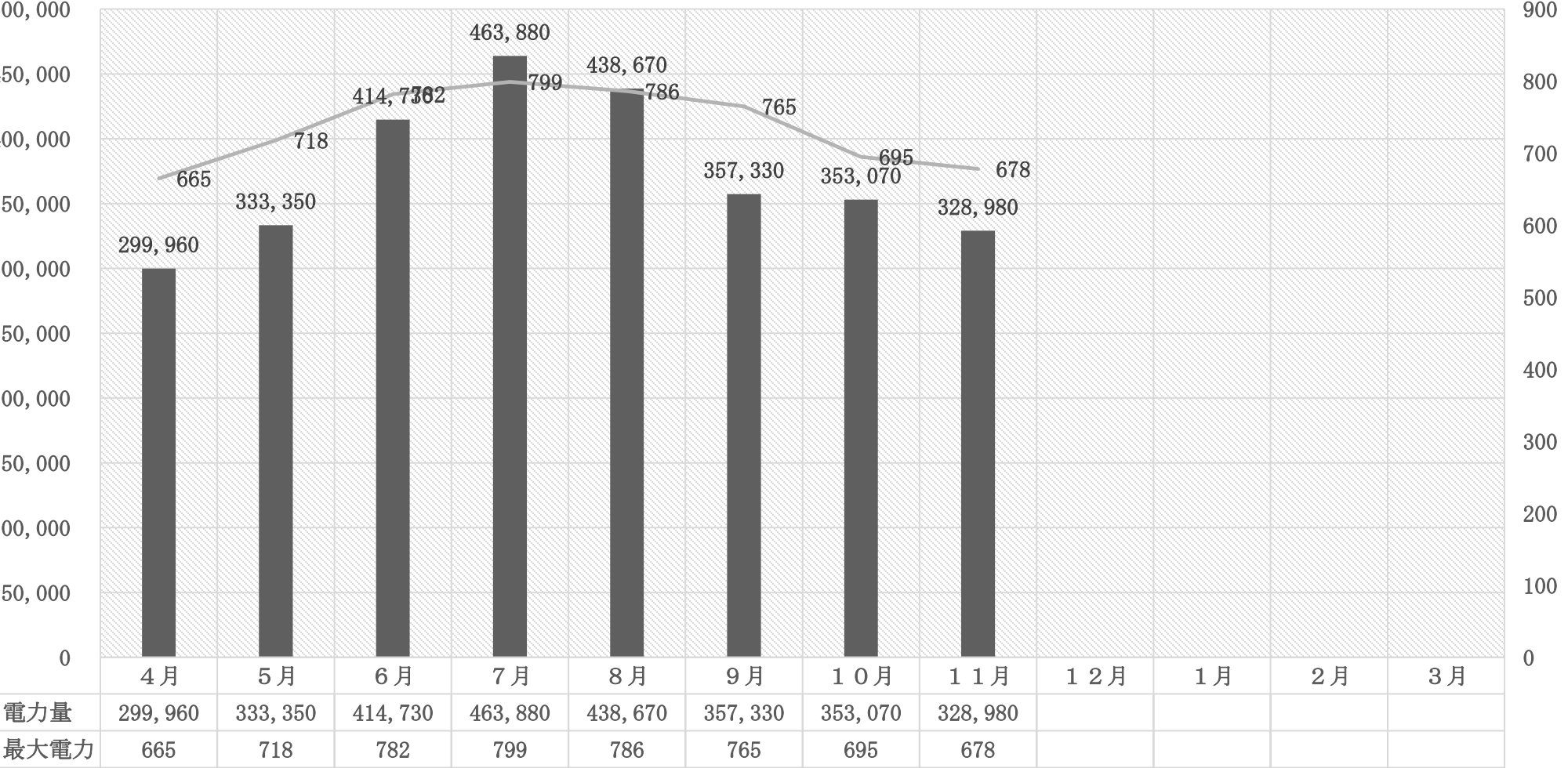
Kwh 令和 4 年度宮古島駐屯地年間使用電力実績表 Kw
