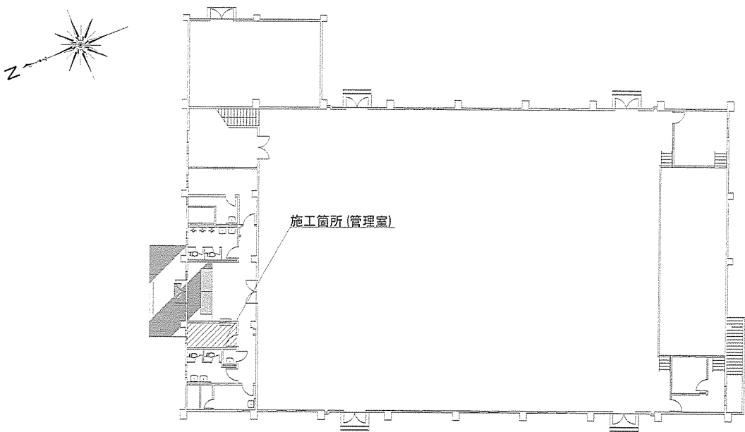
19号建物1階平面図 S=1/300
