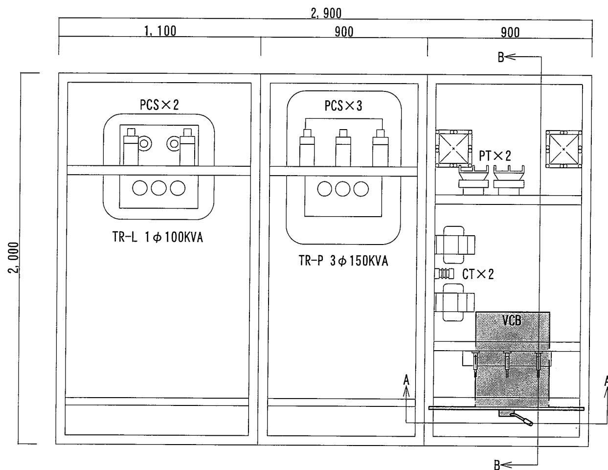
受電設備平面図 S=1/20
