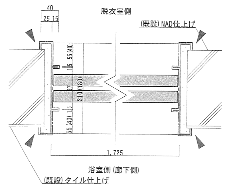
(AD-2・AD-3) A-A断面図 S=1/5
