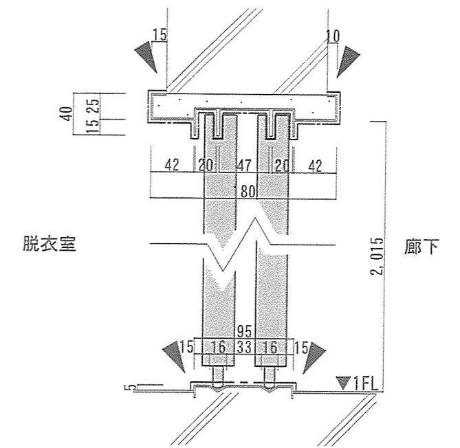
(AD-3) B-B断面図 S=1/5
