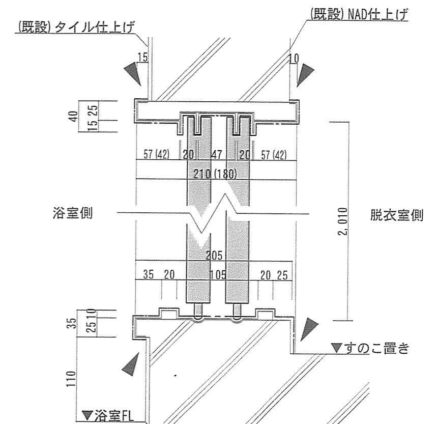
(AD-2) B-B断面図 S=1/5
