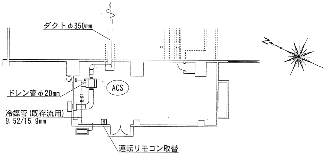
300m射座機械室平面図 S=1/200
