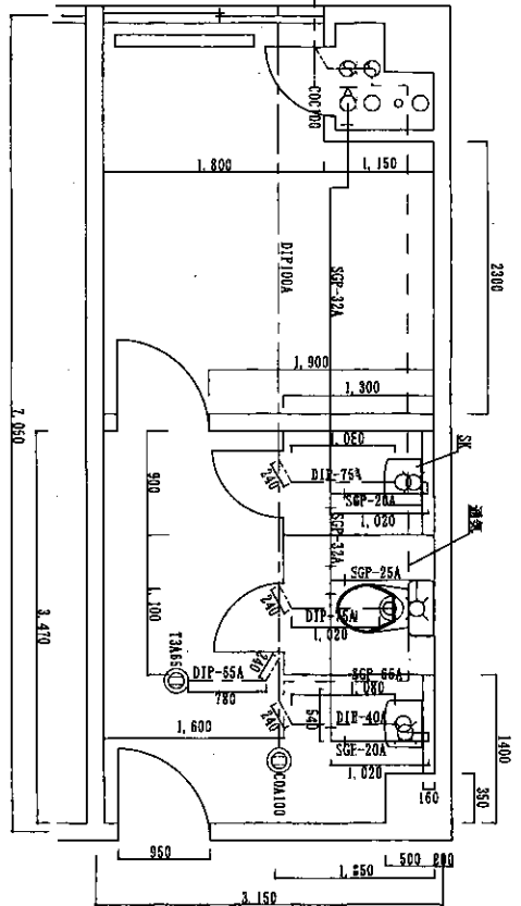
既設平面図 (給排水配管) S=1:60
