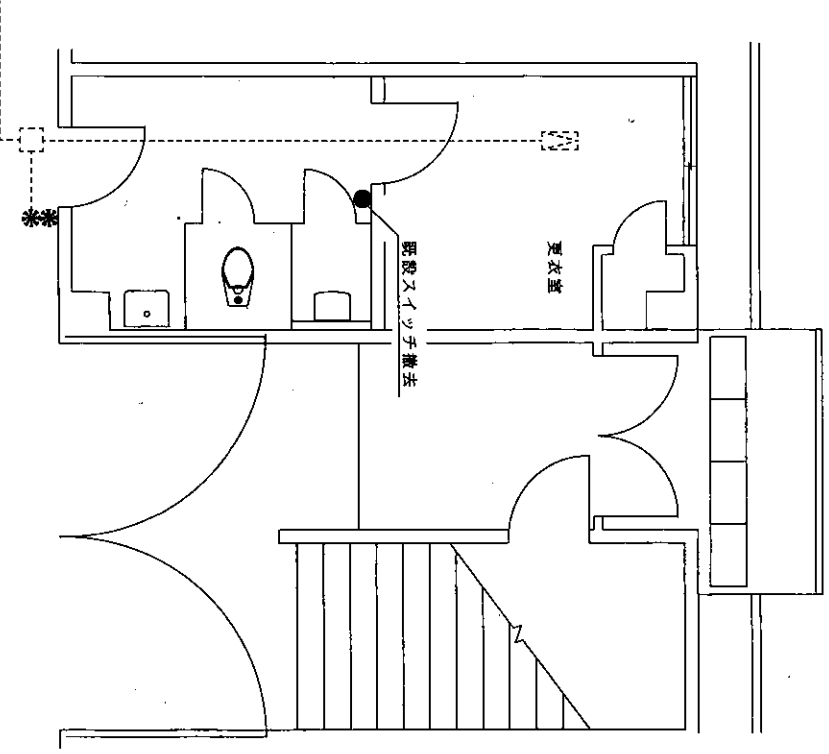
1階女子更衣室等改修前換気線配線図 1/60
