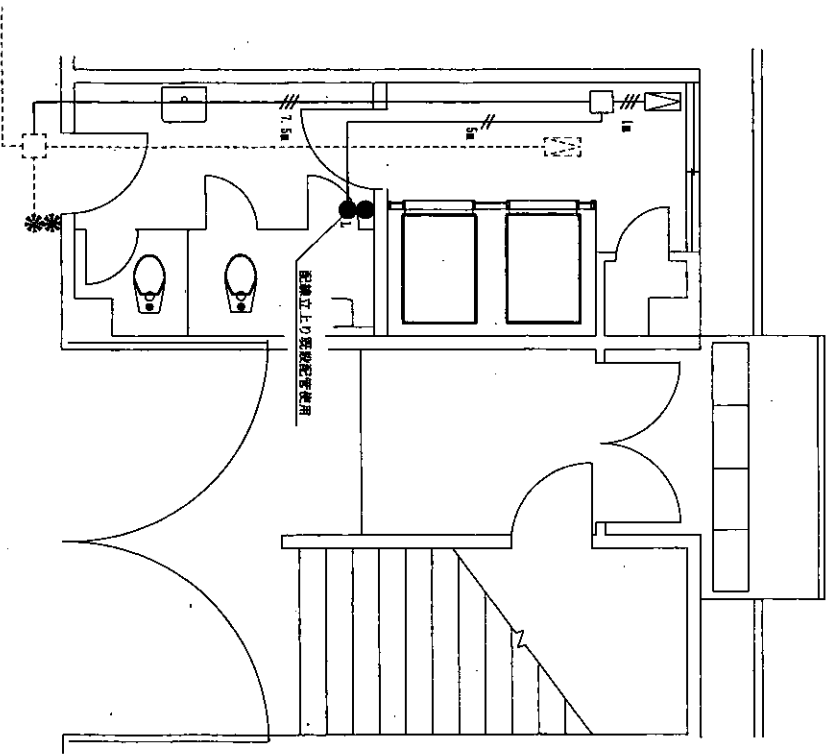
1階女子更衣室等改修後換気線配線図 1/60
