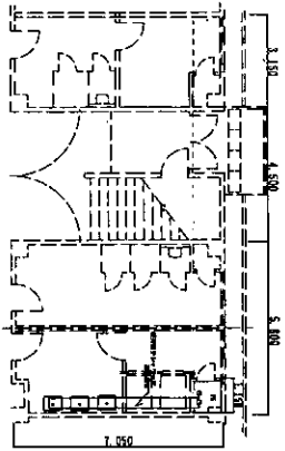
一般隊舎 1階改修前給湯配管平面図 1/200
