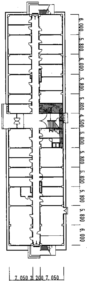
一般隊舎(63号)1階平面図 S=1:4.00
