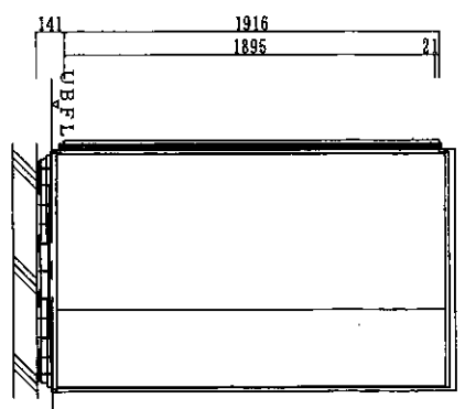
D 展開 S=1/30
