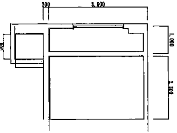
女子更衣室改修前断面図 1/30
