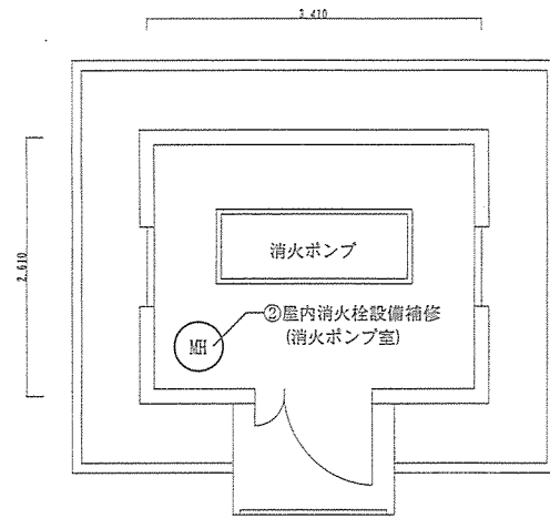
② 249号建物平面図 S=1/60
