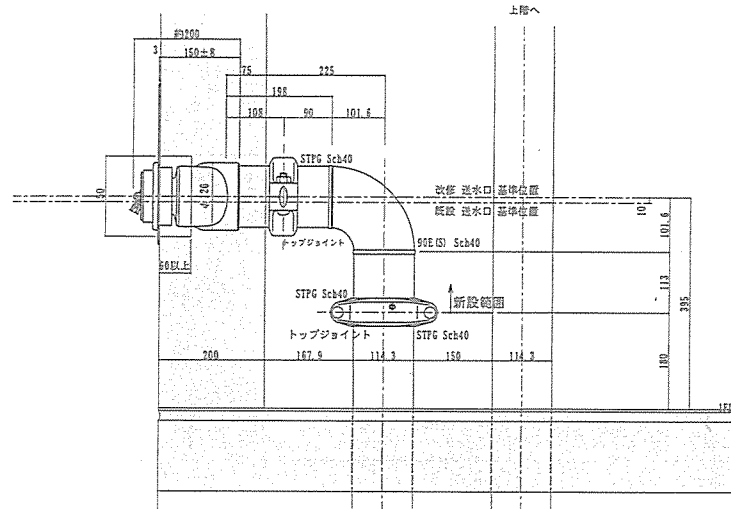
① 連結送水管改修後側面図 (標準) S=1/10
