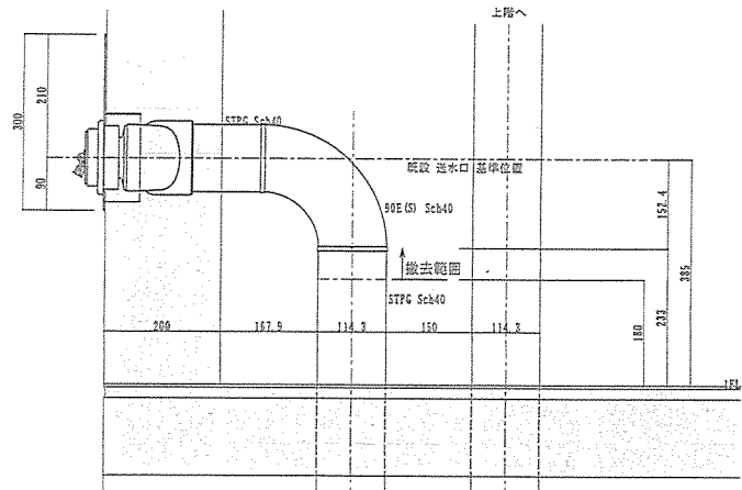
① 連結送水管改修前側面図 (標準) S=1/10
