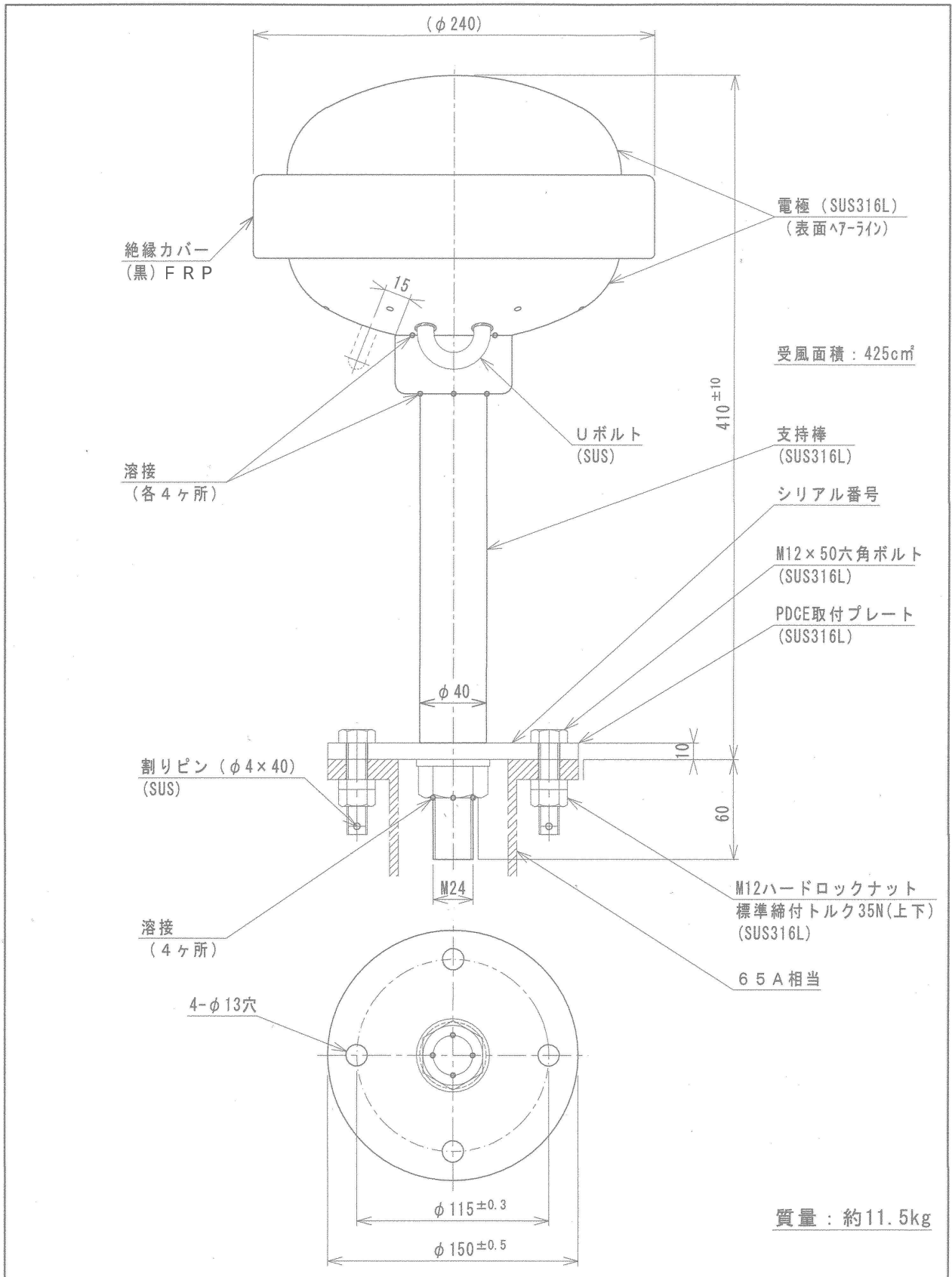
TITLE 国土強靱化対象製品 PDCE-Mg 外観図
