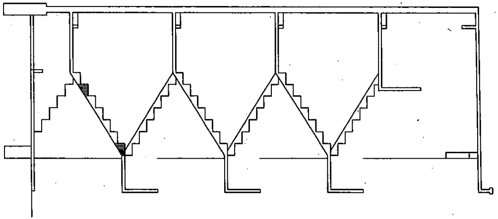
4号棟東側階段施工図
