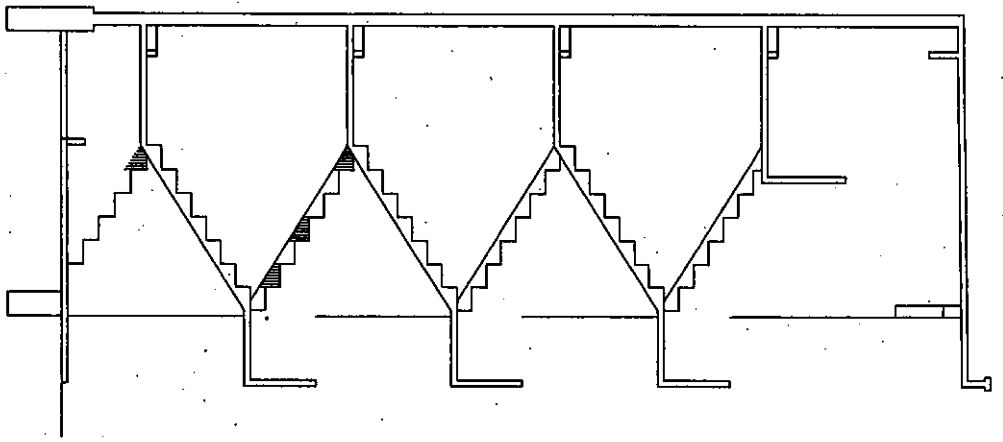
6号棟西側階段施工図
