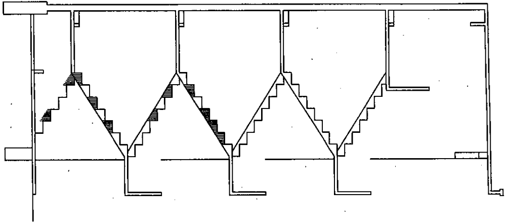
2号棟西側階段施工図
