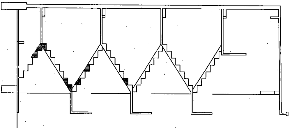
6号棟東側階段施工図
