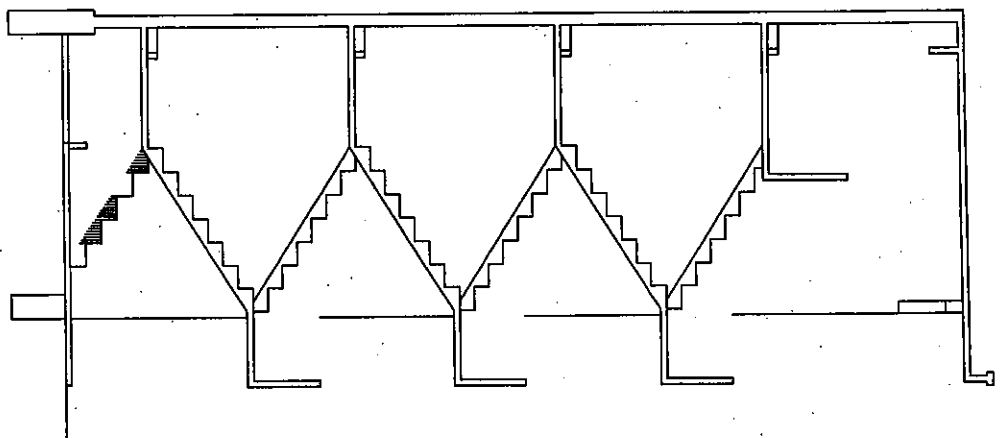
3号棟西側階段施工図
