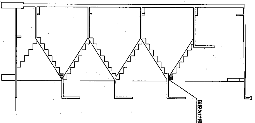
6号棟中央階段施工図
