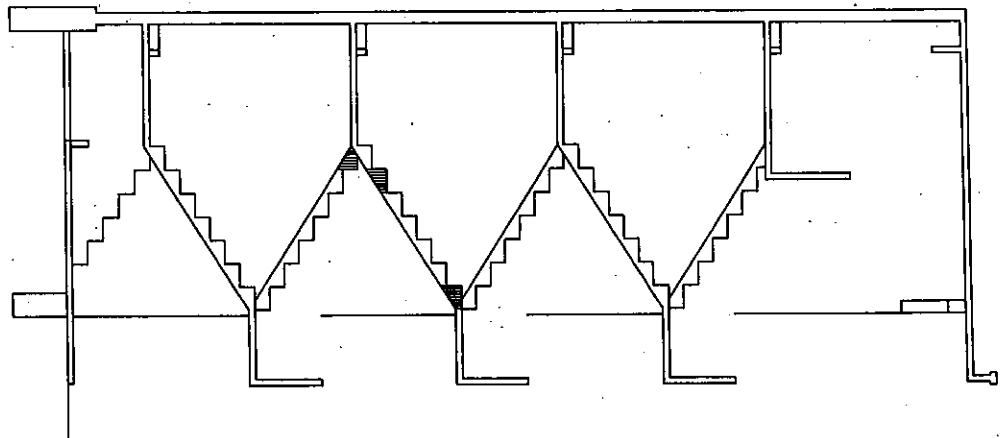
3号棟東側階段施工図
