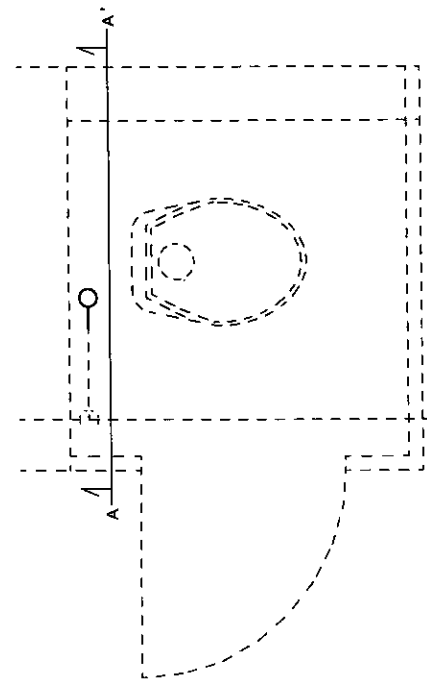
側去基準図 S=1:15
