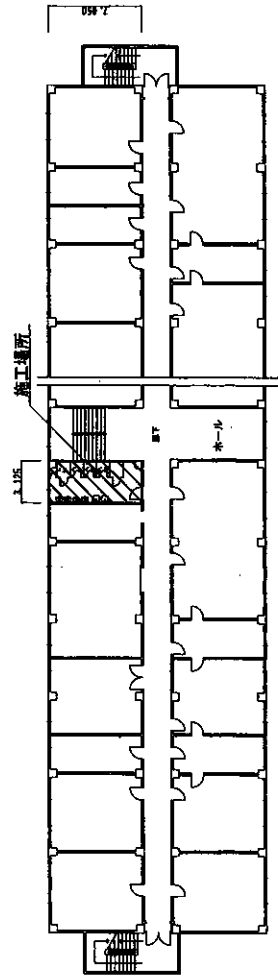
本部兼倉4階平面図 S=1:400
