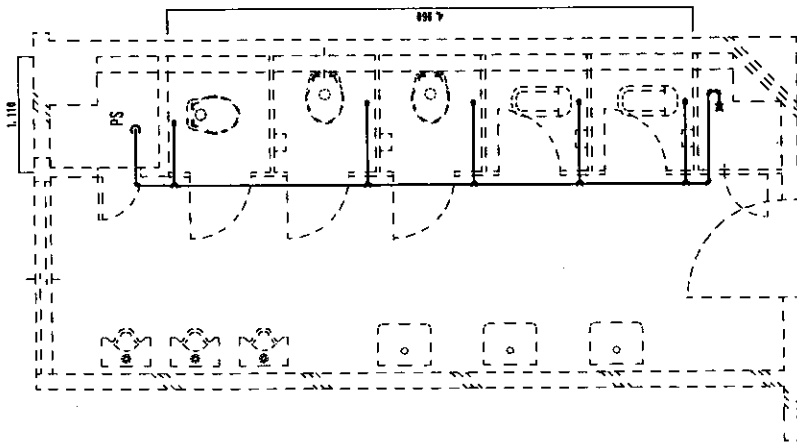
本館階舎4階既設給水管図 S=1:50
