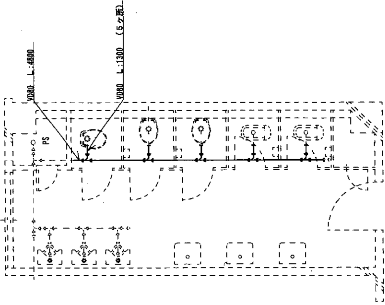
本部階舎4階汚水管施工図 S=1:50
