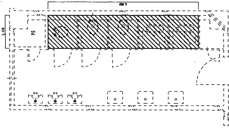
本部兼倉4階施工場所図 S=1:50
