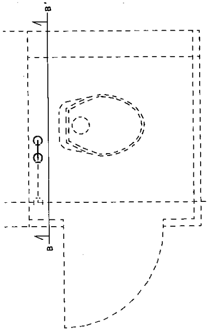
側付基準図 S=1:15
