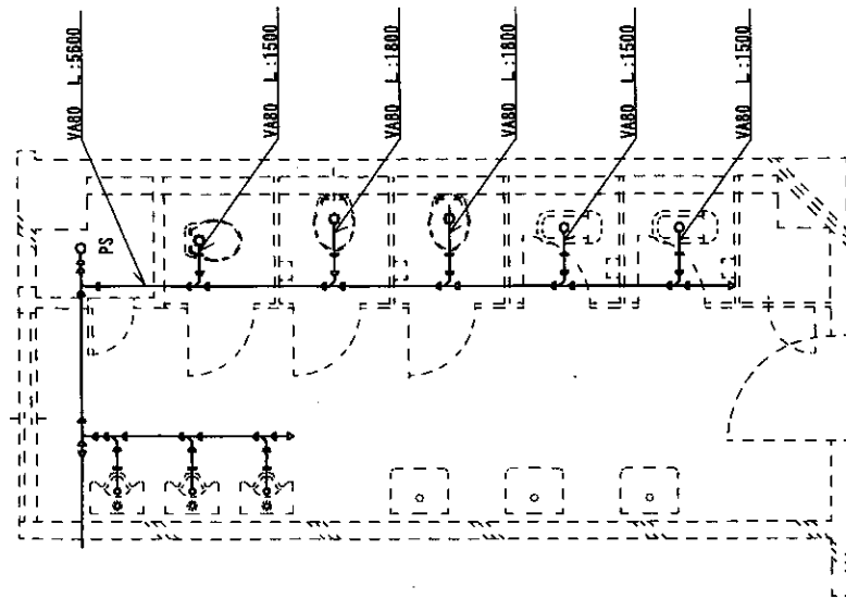
本部階舎4階配汚水管図 S=1:50
