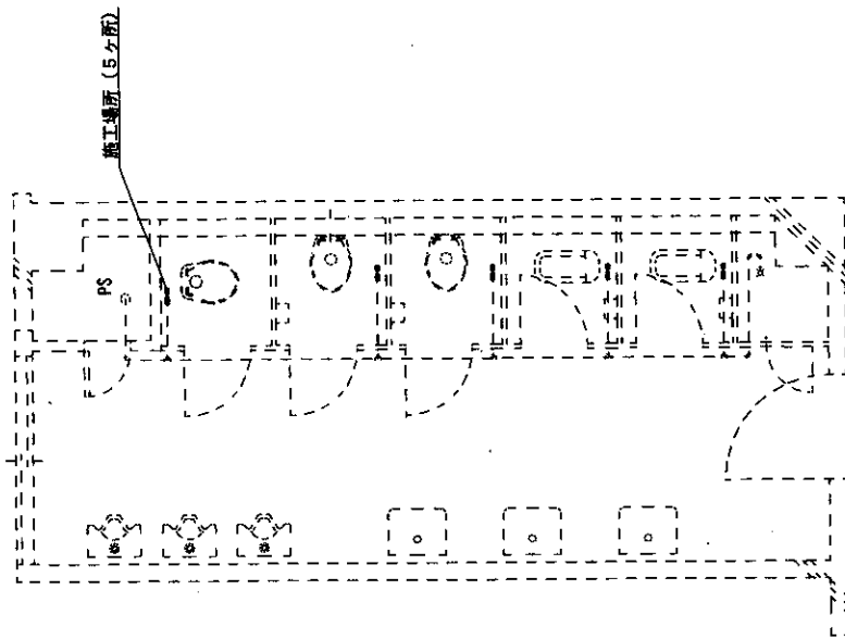
本館階舎4階給水管施工図 S=1:50
