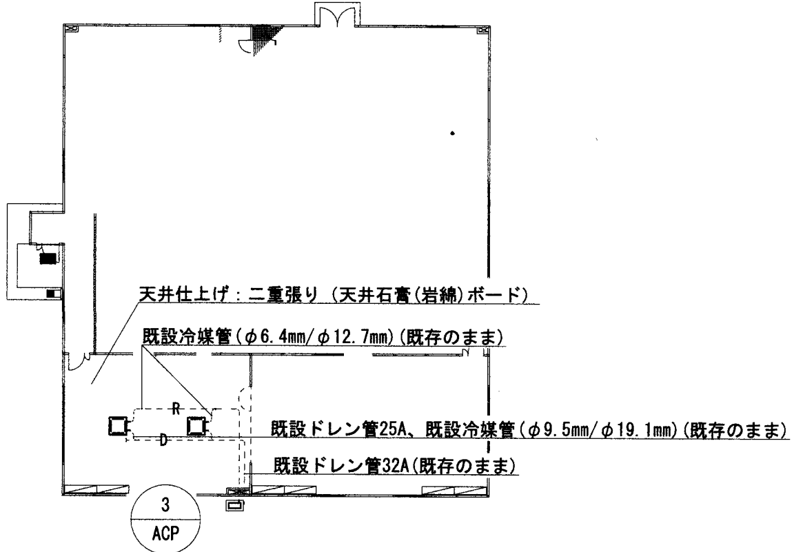
182号建物1階平面図 S=1/300
