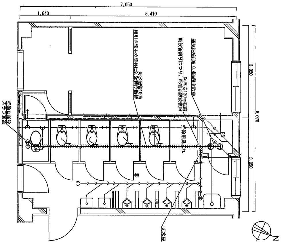
1号建物 2 F 便所平面图 S=1:50
