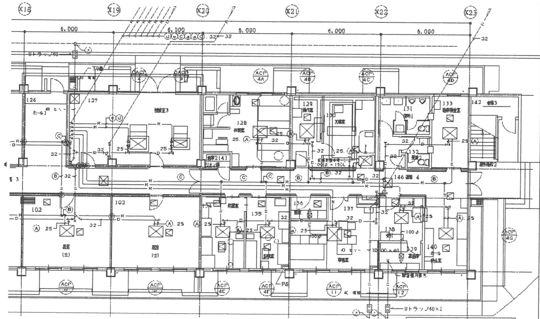
隊舎 1階 平面図 (配管) S=1/150
