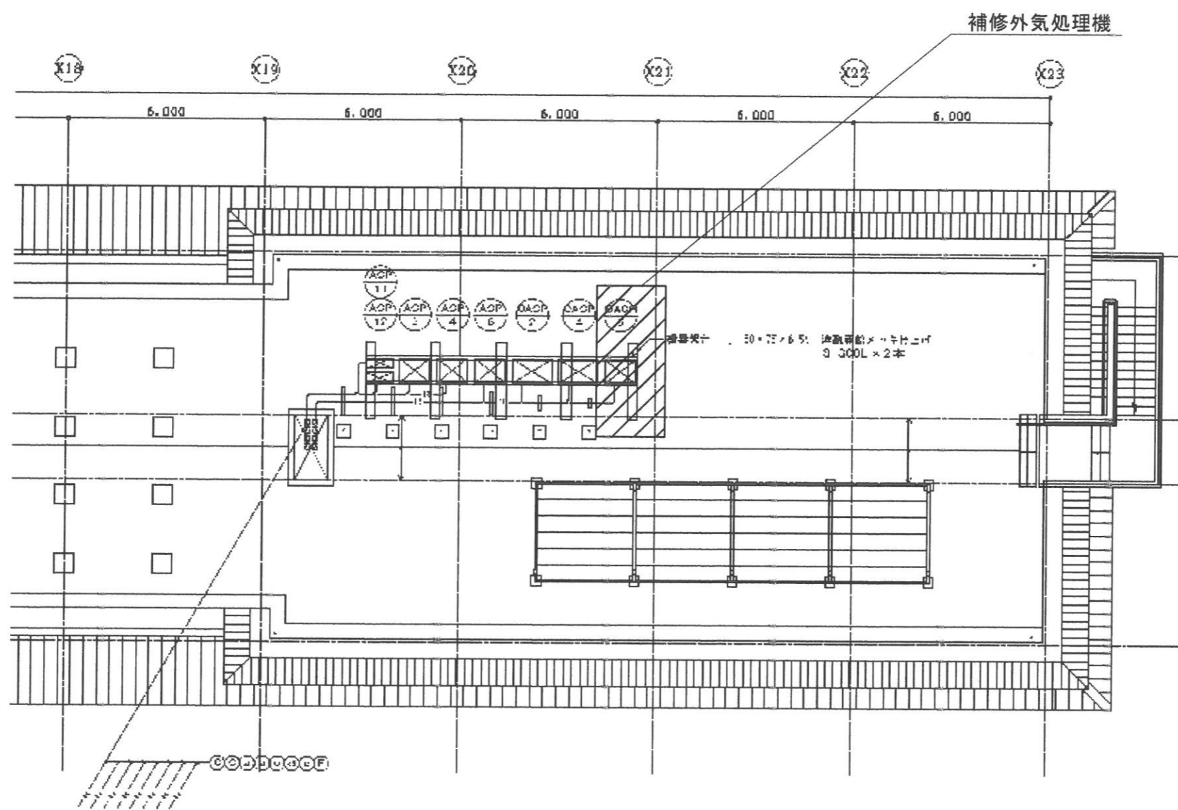
隊舎 R階 平面図 S=1/600
