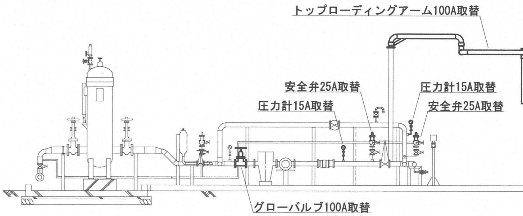
B ~ B' 立面図 S=1/60
