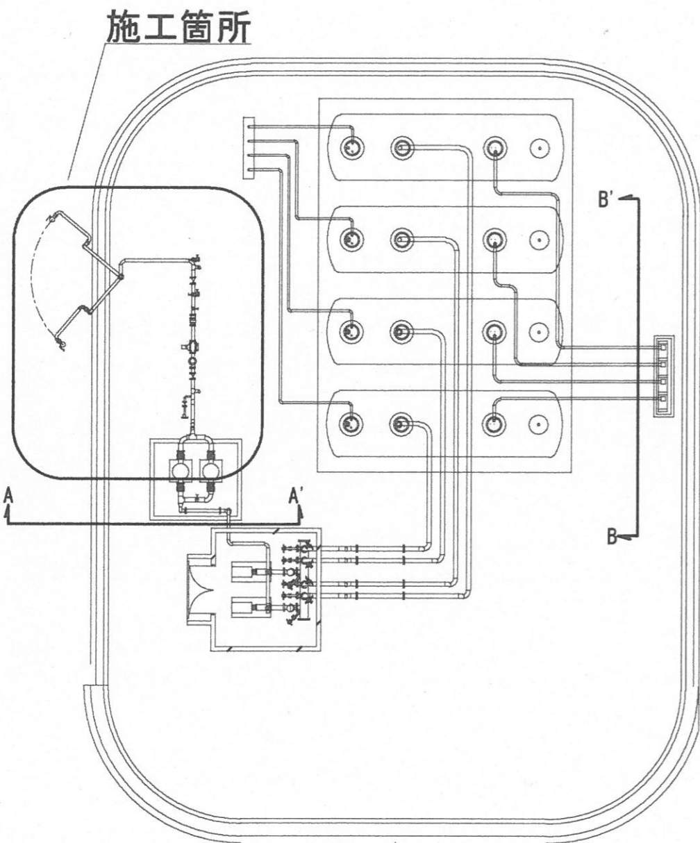
燃料施設 平面図 S=1/200
