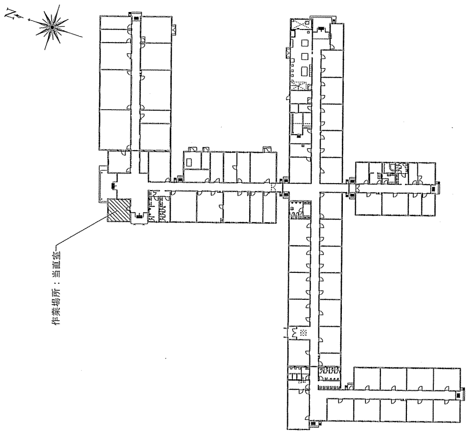
隊庁舎平面図 S=1/600
