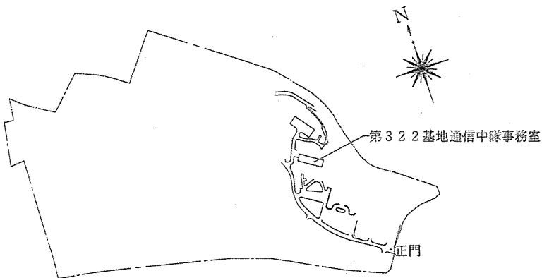
那覇駐屯地配置図 S=1:X
