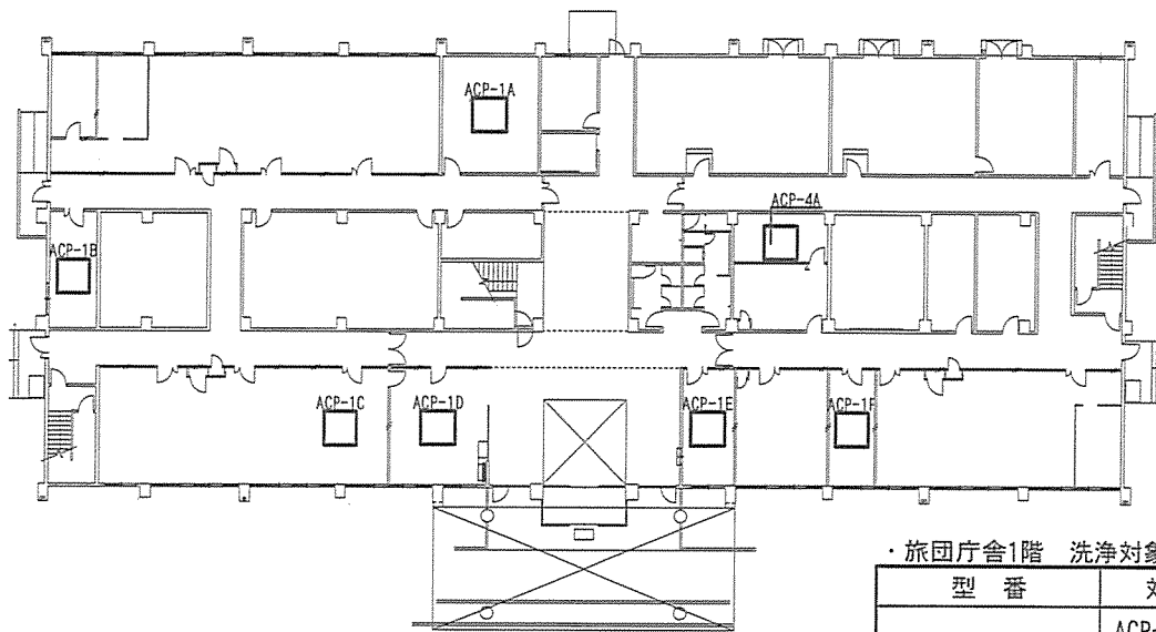
旅団庁舎1階平面図 S=1/500
