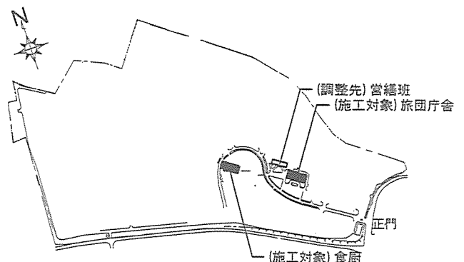
配置図 S=1/8,000
