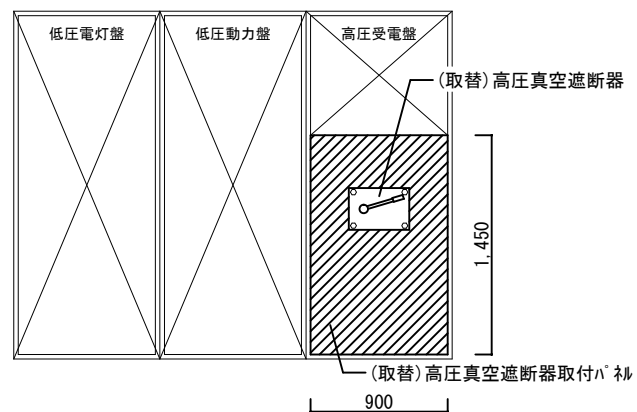
受電盤立面図 S=1/50
