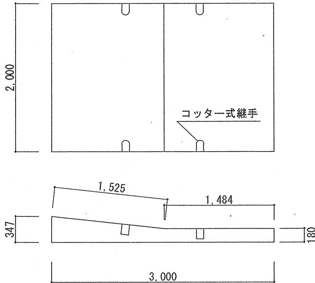
枕版標準図 S=1/50
