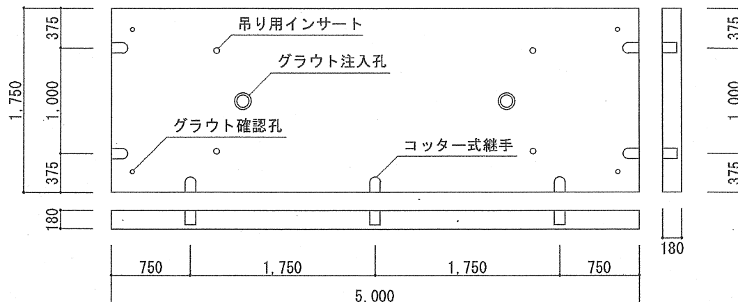
道路用 P R C 版 ( A ) 標準図 S=1/50
