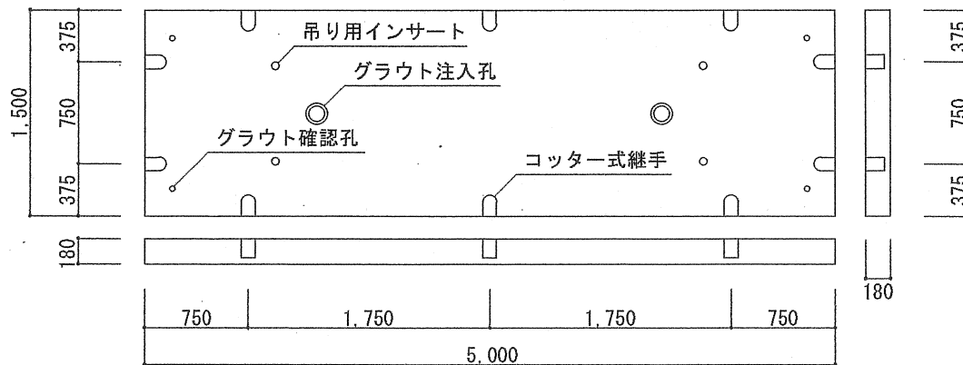
道路用 P R C 版 ( B ) 標準図 S=1/50
