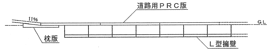
施工計画断面図 S=1/200
