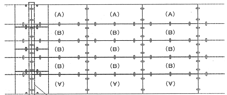
施工計画断面図 S=1/200
