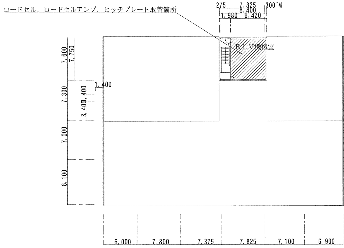
補給倉庫 R F 階平面図
