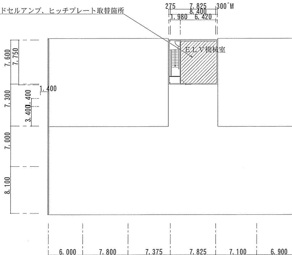
補給倉庫 R F階平面図
