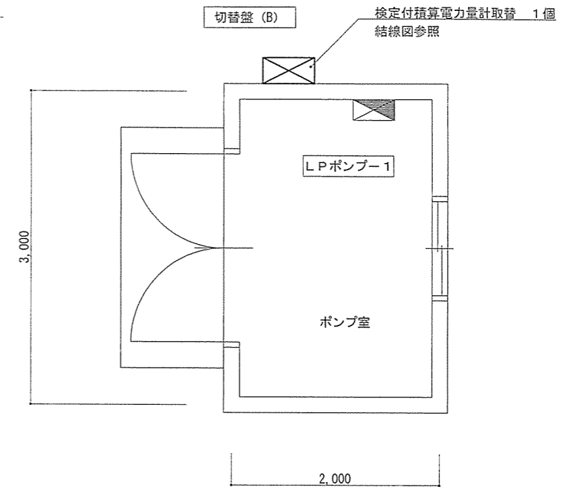
67号建物 動力幹線設備 平面図 S=1:50
