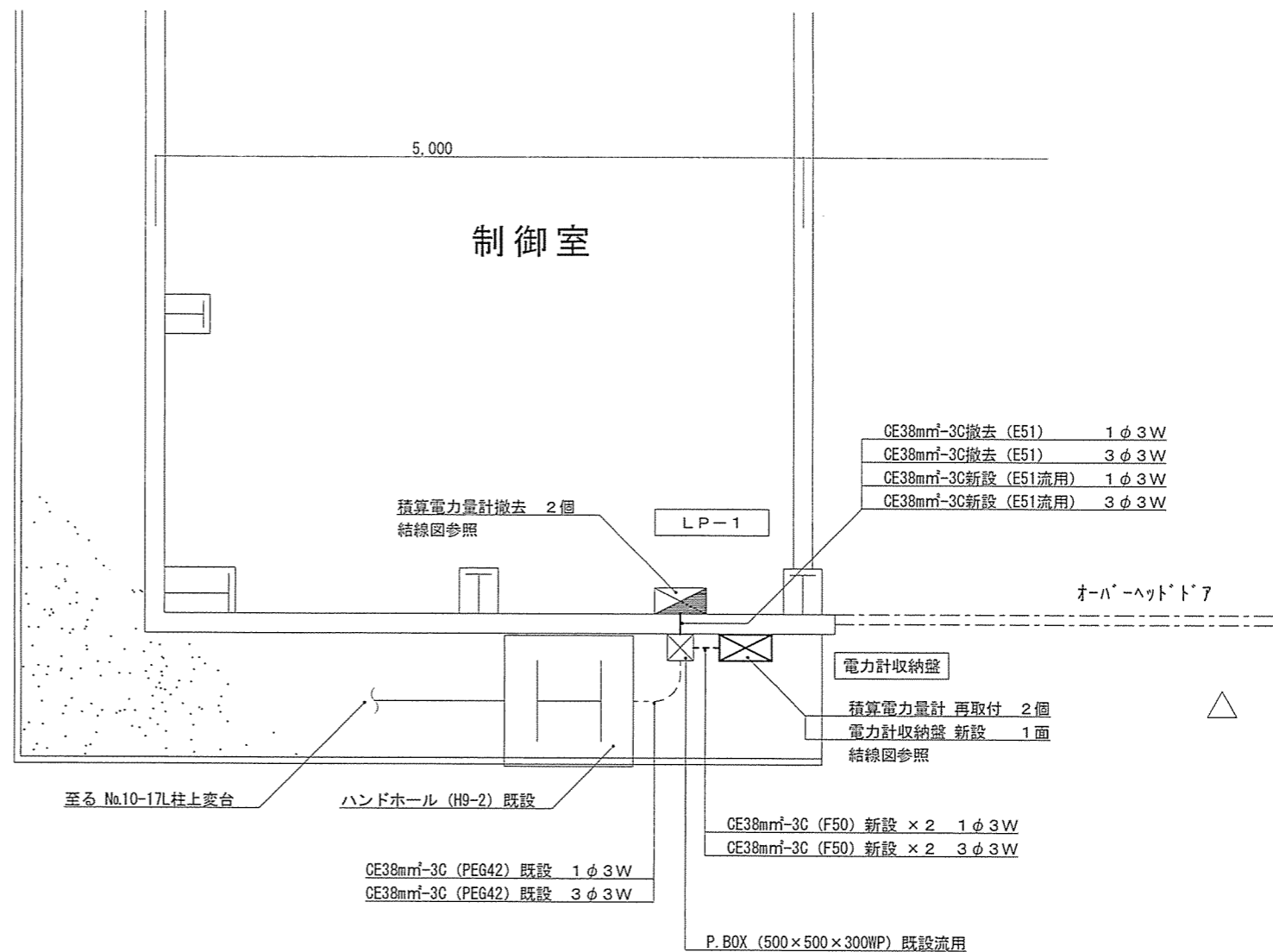
579号建物 動力幹線設備 平面図 S=1:50
