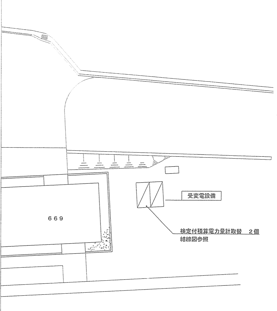
669号建物 受変電設備 配置図 S=1:200
