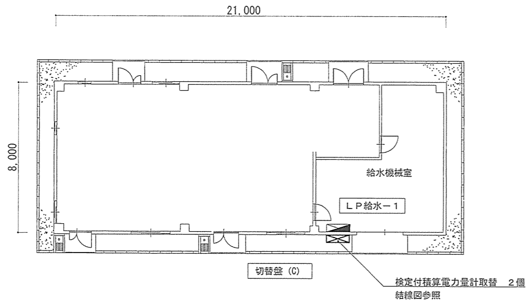
66号建物 動力幹線設備 平面図 S=1:200
